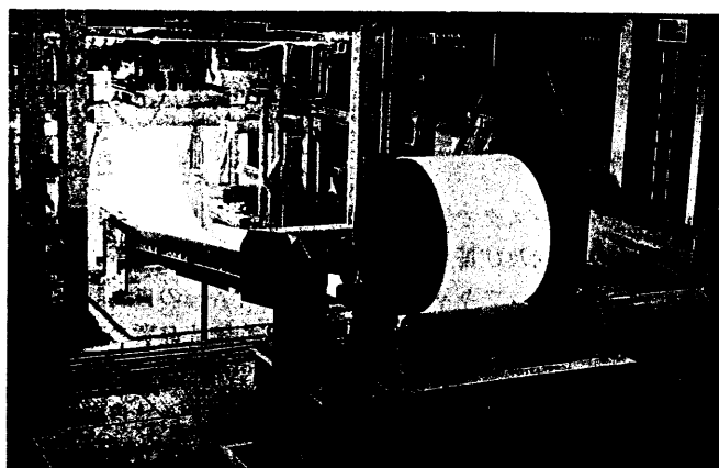
図1 600 mm 幅ストリップキャスト試験機 casting 状況 ストリップキャスト試験機によるステンレス鋼の casting 状況。 Casting condition of 600 mm wide strip caster
