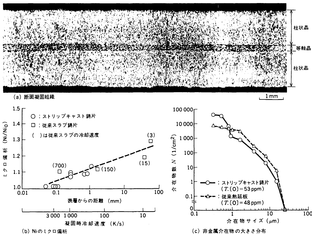
図5 ストリップキャスト鑄片特性 ストリップキャスト鑄片の(a)断面凝固組織、(b)Niのマイクロ偏析及び(c)非金属介在物の大きさ分布を示す図。 Characteristics of cast strips
