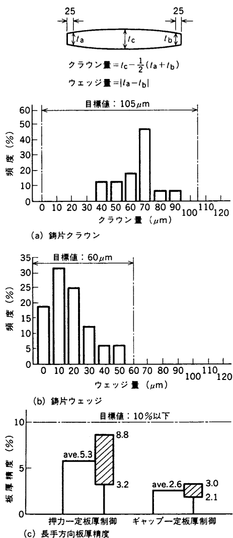
図6 ストリップキャスト鋳片の形状 ストリップキャスト鋳片の (a) クラウン量, (b) ウェッジ量及び (c) 長手方向板厚精度を示す図。 Cast strip profile
