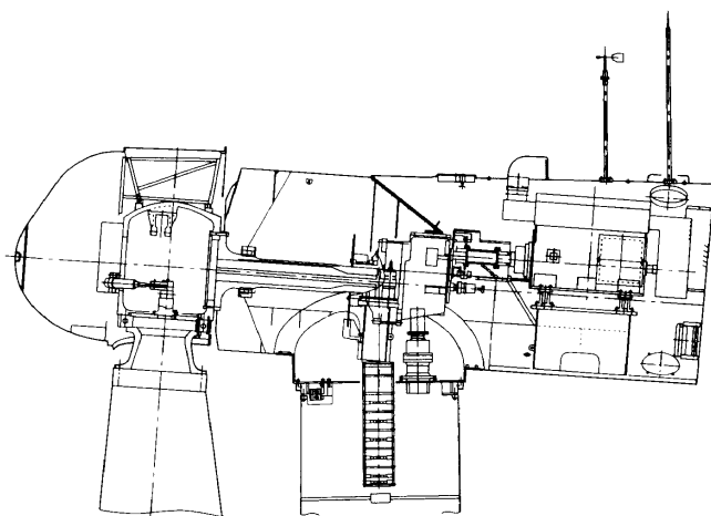
図2 ナセル構造 MWT-1000に採用した軽量ナセル及びナセル内構造を示す。 Nacelle of MWT-1000
