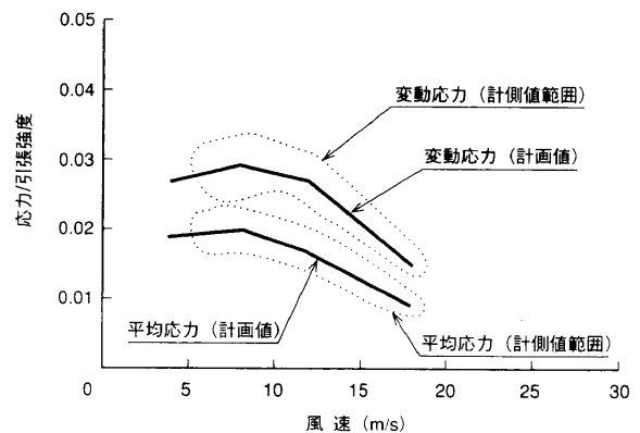
図7 主軸応力計測結果 風速に対する主軸応力の計測結果を示す。 Result of main shaft stress measurement
