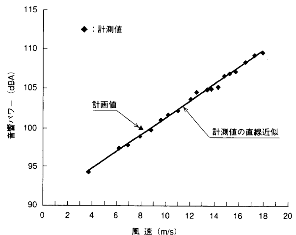
図8 騒音計測結果 風速に対する音響パワー計測結果を示す。 Results of noise measurement
