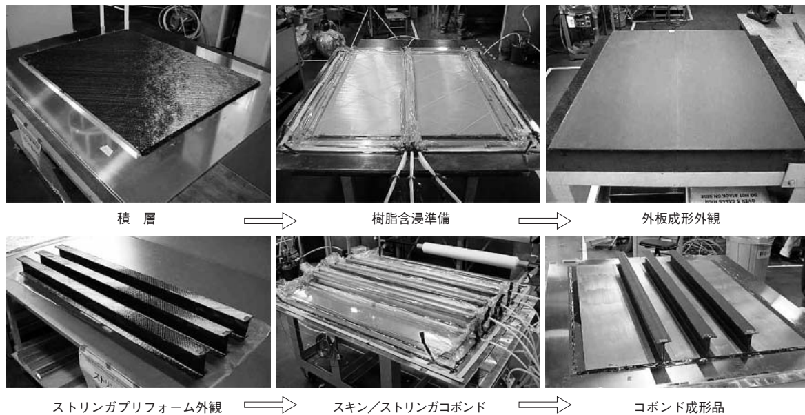
図5 3ストリングパネル成形工程
