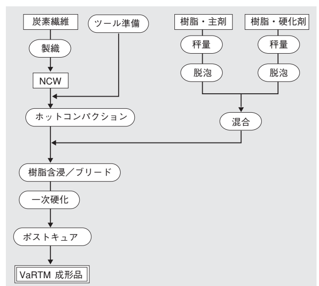
図3 A-VaRTMによる複合材成形フロー
