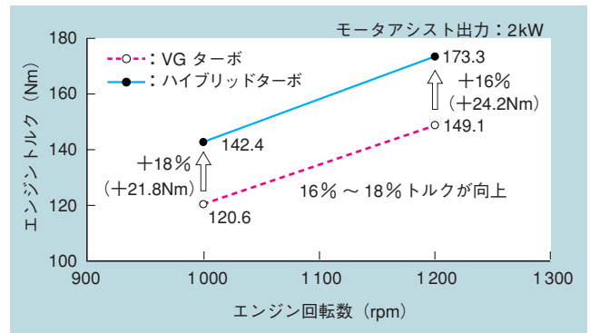
図7 ハイブリッドターボとVGターボのエンジン定常トルク比較 モータアシストによりエンジン低速時に16-18%のトルク向上が得られる。
