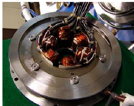
図5 ハイブリッドターボの試験状況及びモータステータ外観 エンジン試験中のハイブリッドターボ。モータステータは6スロット集中巻きで低損失小型化を図った。
