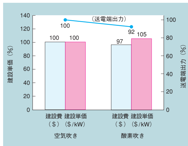
図3 CO 2 回収時の空気吹きと酸素吹き IGCC における建設費及び建設単価と送電端出力の比較
