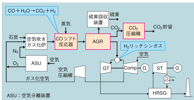
図2 CO 2 回収時の空気吹き IGCC システム概略系統図
