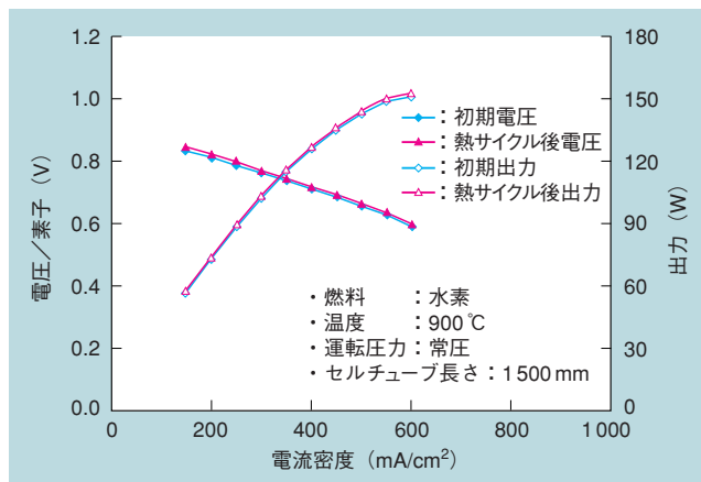
図 4 高出力セルチューブの電流／電圧特性 高出力セルチューブにて最大定格出力 151 W を確認。
