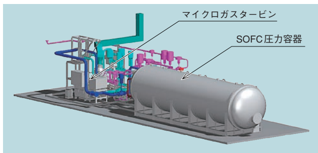
図 1 200 kW 級 SOFC-MGT コンバインドサイクルシステム マイクロガスタービンとの組合わせによる世界最大級の加圧コンバインド発電システム。
