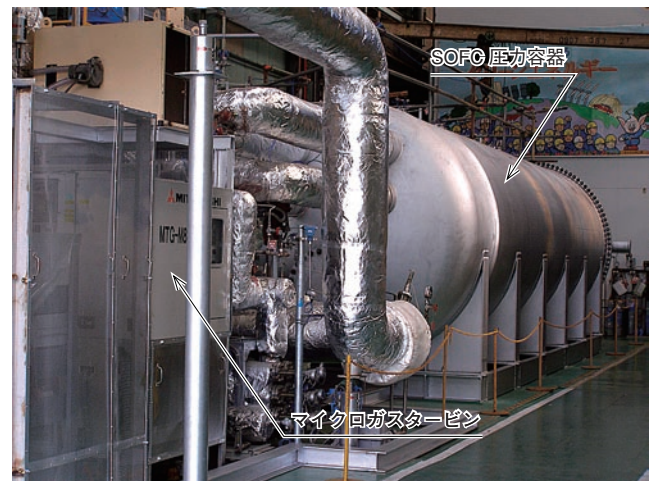
図8 200 kW 級 SOFC-MGT コンバインドサイクルシステム外観図
