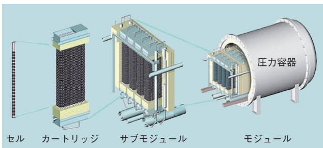
図6 モジュール構成
