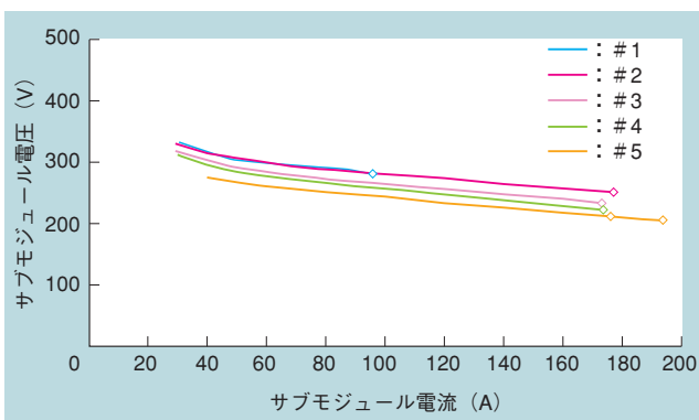
図7 改良型モジュールの単体性能
