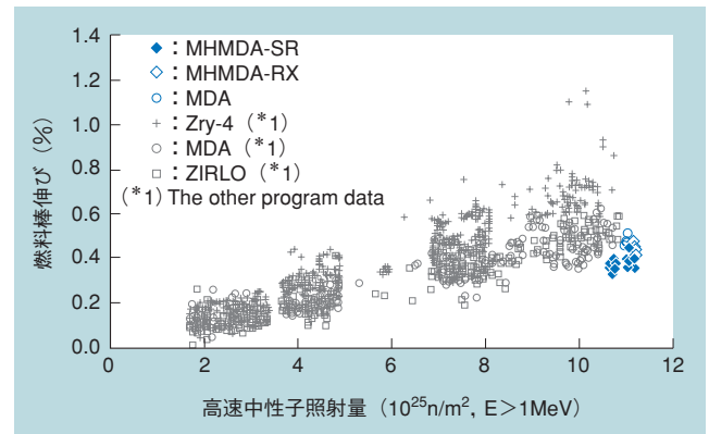
図5 燃料棒伸び
