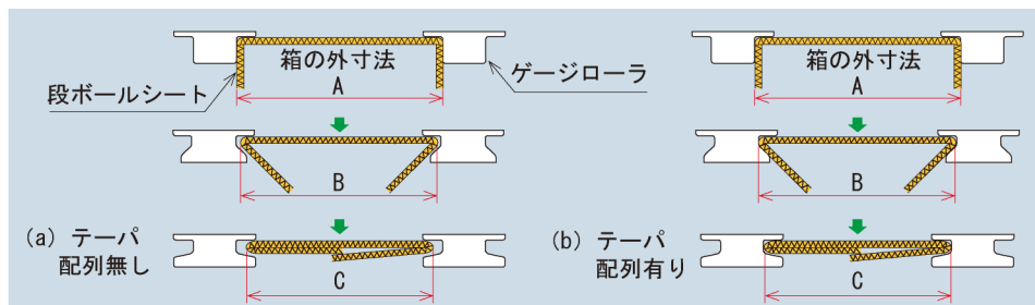
図4 可変テープ配列ゲージローラ装置概念図(シート進行方向断面図)
