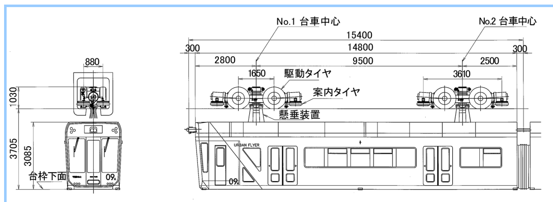
図1 形式図
