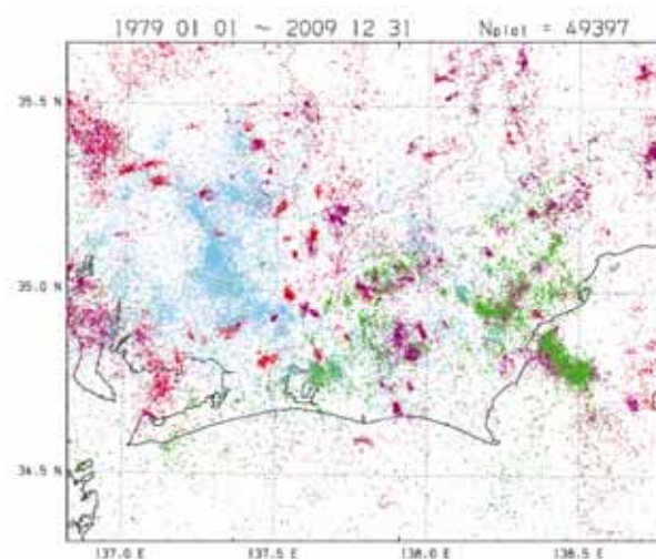
図 4 東海の微小地震分布。色分けは、震源の深さに対応し、赤が浅く、青が深い。
