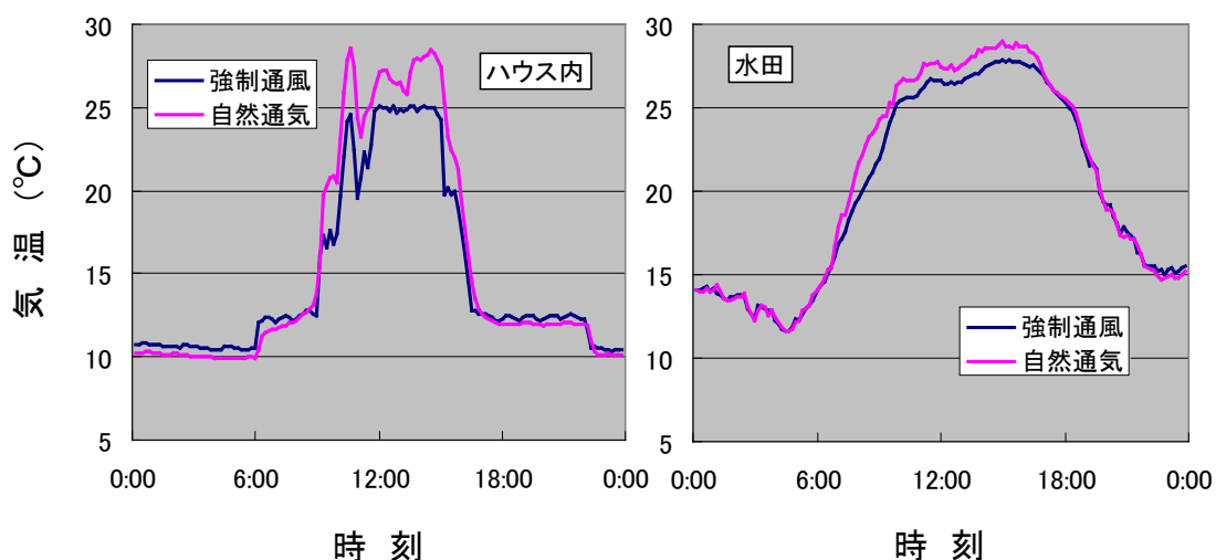
図 3. 強制通風式放射よけと自然通気式放射よけによる気温計測値の比較. 左:プラスチックハウス内, 右:水田
