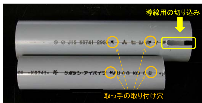
図 11. 塩ビ薄肉管の加工. 50A×25 cm(上), 40A×20 cm(下)
