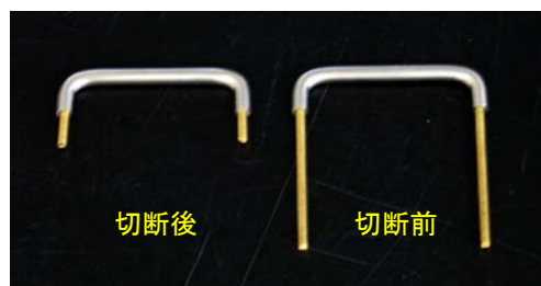
図 9. 取っ手のネジを 10 mm に切断
