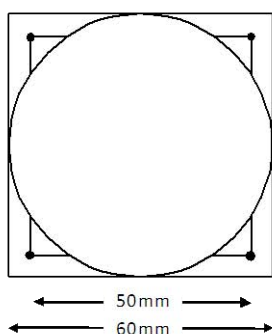
図 7. ファン取り付け穴 用ガイド. ●が穴位
