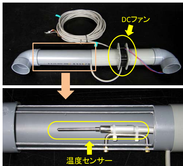
図 4. 完成品(上)とセンサー取付部のカットモデル(下)
