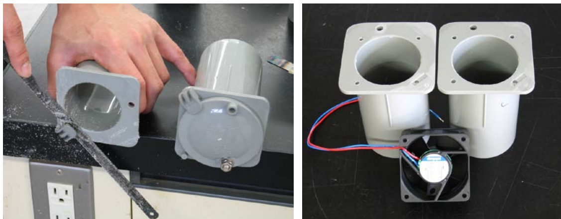
図 6. 分水栓の加工. 不要部分を切り落とし(左), ファン取り付け穴を開ける(右)
