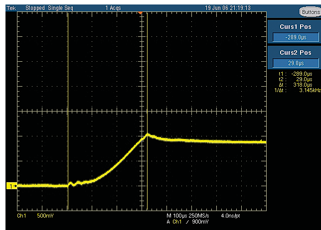
図 2 シンクロトロンのビーム電流の側定例（100 \mu s/div.）。ビームがリニアックからリングに入射されたところで、多重入射でリング内のビーム電流が約 200 \mu s で増えているのがハッキリと測定できる。
