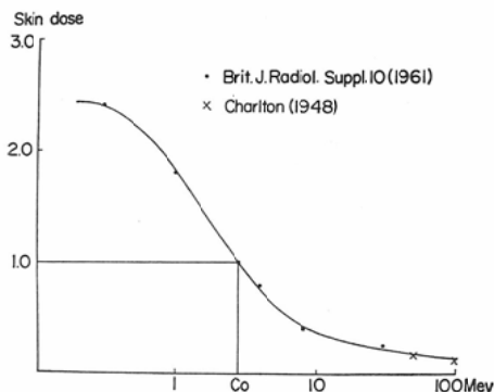
図2： ^{60}\text{Co} \gamma 線の入射皮膚線量を1とした場合の，他のエネルギーのX線の皮膚線量。
