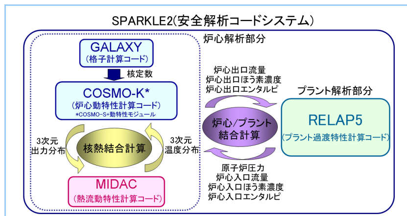
図1 Non-LOCA 安全解析コードシステム SPARKLE2 の全容
