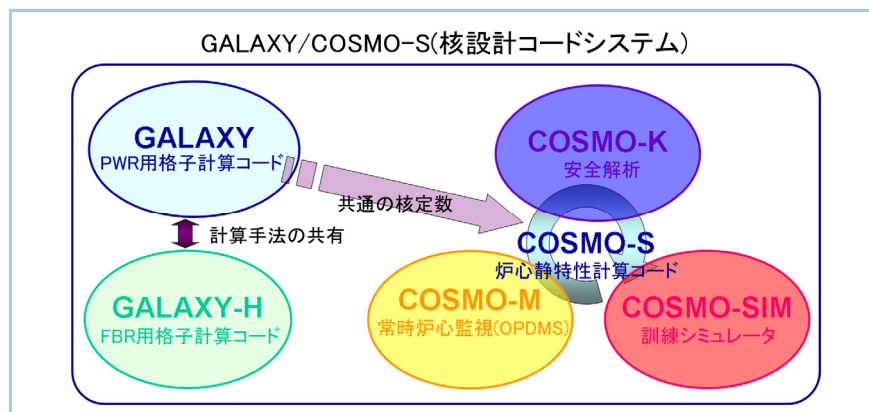
図2 核設計コードシステム GALAXY/COSMO-S の全容とインターフェイス
