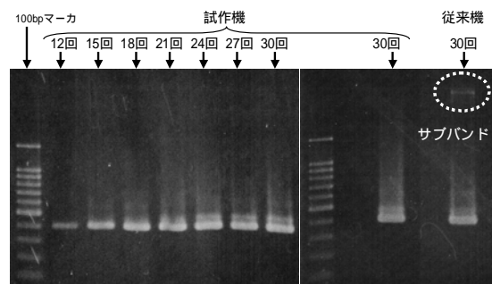
図10 試作機および従来機(ペルティエ式)のPCR実験結果
