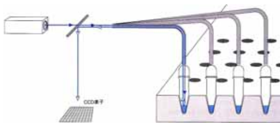
図2 従来のペルティエ式 PCR 装置の測定原理
