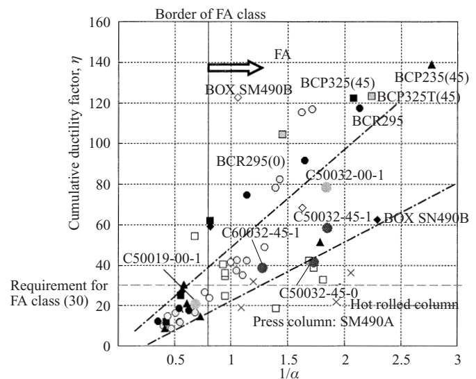
図 3 累積塑性変形倍率 \eta - 無次元化幅厚比 \alpha 関係
