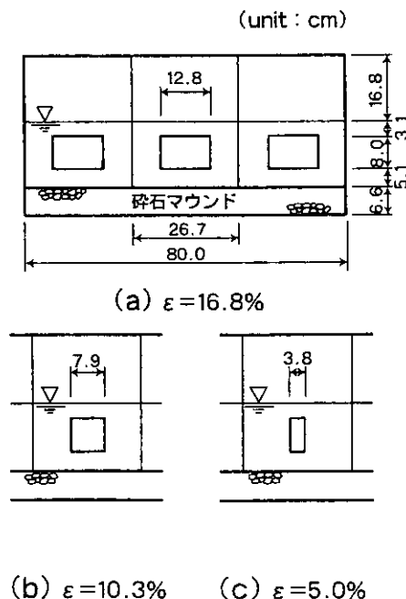
図-4 堤体模型正面図
