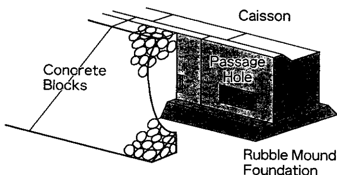
図-1 消波ブロック被覆型有孔堤の概念図
