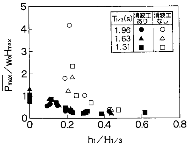
図-7 孔内波圧に及ぼす孔水深の影響
