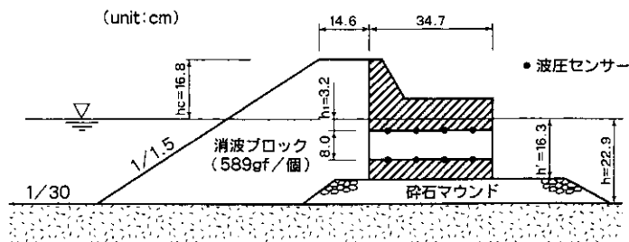
図-3 堤体模型の基本断面
