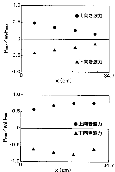
図-6 通水孔内の波圧分布例 ( T_0=1.96\text{s} , H_0'=21.3\text{cm} )
