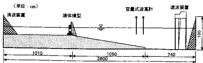
図-2 実験水路
