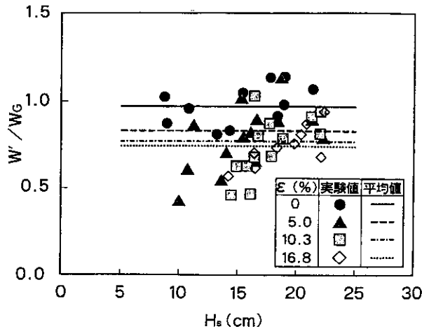
図-8 滑動波力に及ぼす開口率の影響
