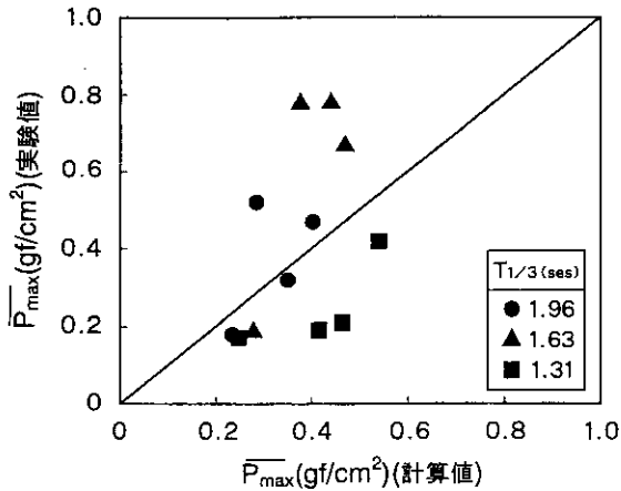
図-10 通水孔内揚圧力の計算値と実験値の比較
