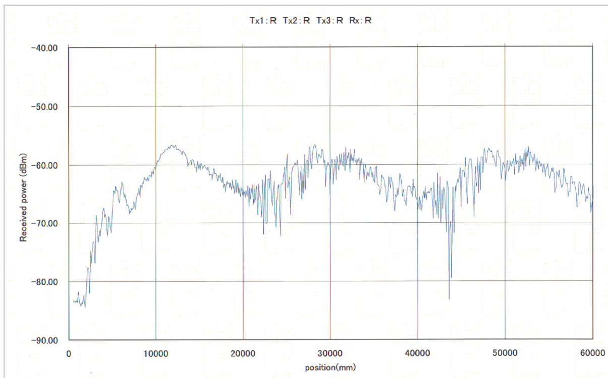
図8 受信電力の測定値 基地局の位置は0, 20, 40m
