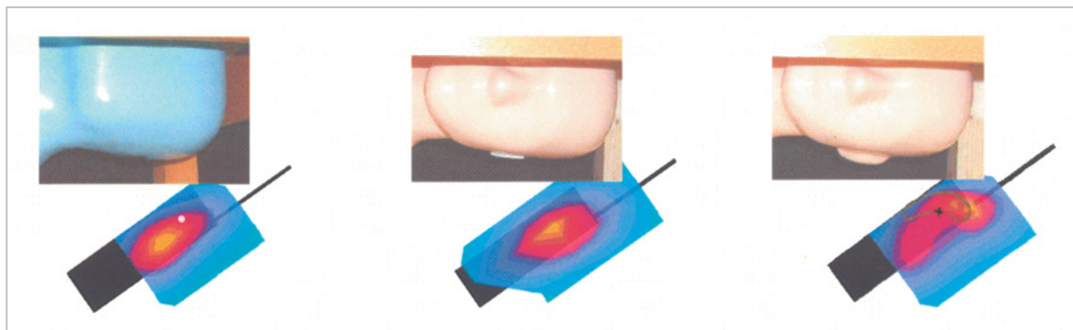
図1 ファントムSAR分布 欧米人モデル(左)、日本人モデル(無損失耳翼、中央)、日本人モデル(損失性耳翼、右) 周波数900 MHz アンテナ放射電力を1 Wに規格化
