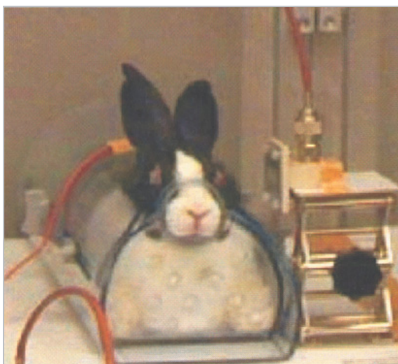
図8 パルス波曝露装置 開口導波管 周波数 2450 MHz
