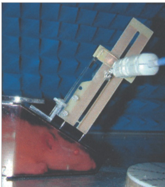
図7 ラット脳曝露装置 微小ループ 周波数 1500 MHz
