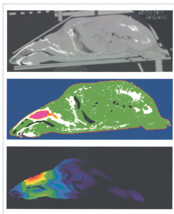
図9 ラット MRI 画像(上)、数値モデル(中)、SAR 分布計算結果(下) 微小ループアンテナ 周波数 1500 MHz
