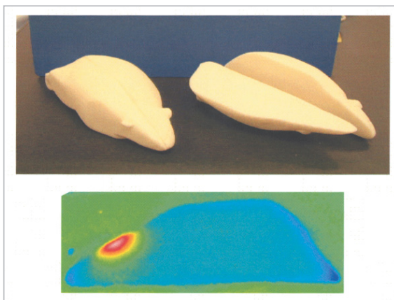
図10 固体ラットファントム(上) SAR分布測定結果(下) 微小ループアンテナ 周波数1500 MHz
