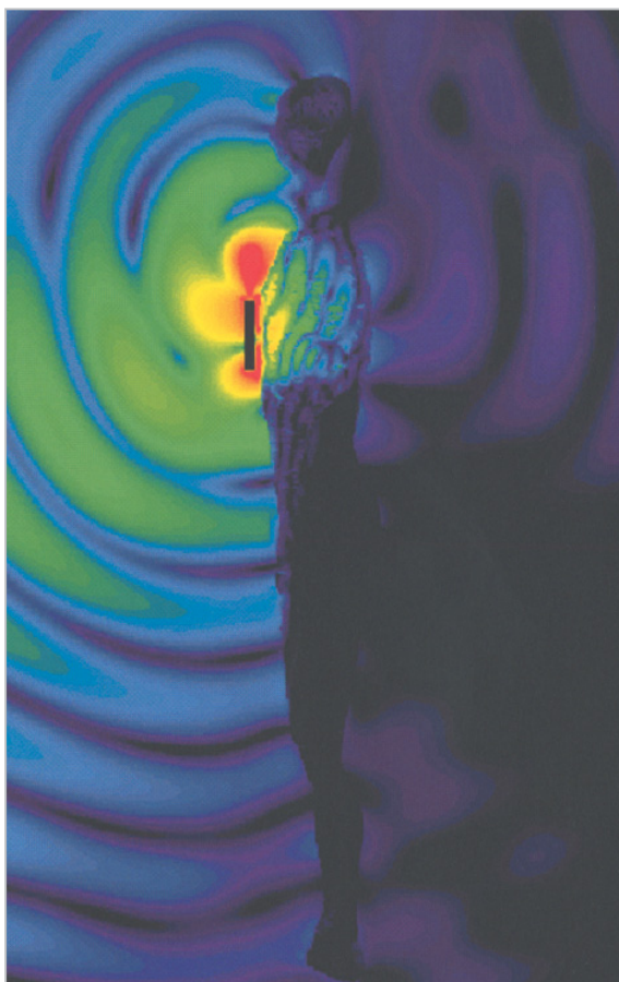
図 12 全身数値モデル(男性)の胸前面の携帯電話による電界強度分布 周波数 900-MHz
