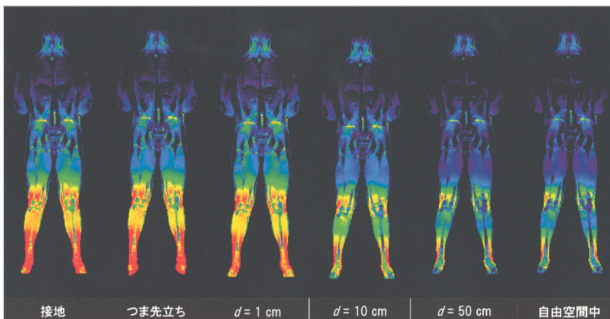
図3 様々な接地条件下での人体垂直断面 SAR 分布 E 偏波平面波入射 周波数 40 MHz(大地上人体の共振周波数付近)
