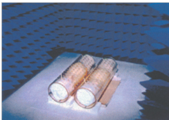
図4 ラット肝臓局所曝露装置 共振長モノポールアンテナ 周波数900 MHz 1500 MHz
