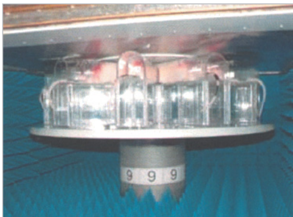
図6 長期実験用ラット脳局所曝露装置 共振長モノポールアンテナ 周波数1500 MHz
