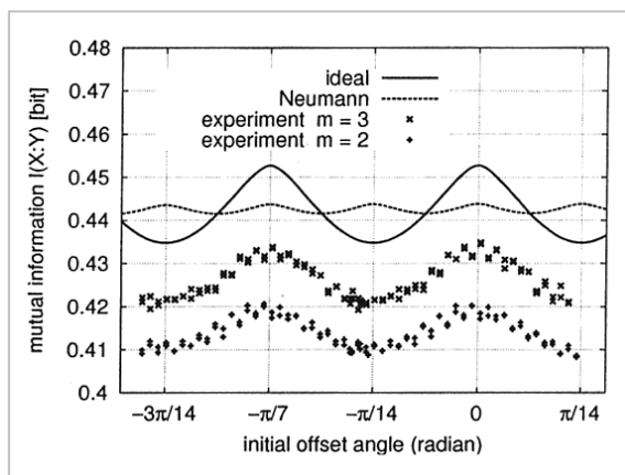
図 11 7元信号の場合の相互情報量の \theta_0 依存性。
