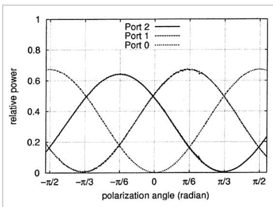
図7 三つのAPDでの相対出力強度。3元信号の場合
