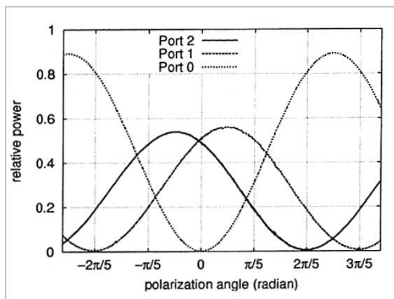
図9 5元信号の場合の三つのAPDでの相対出力強度
