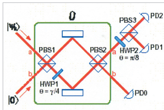
図4 最適POMを実現する検出回路の概念図
