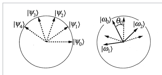
図6 測定ベクトルと信号ベクトルの間に加える相対角 \theta_0 。M=5の場合の図。
