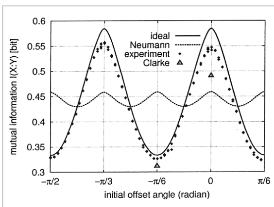
図8 相互情報量の \theta_0 依存性。3元信号の場合 + が実験値、実線が理論値、点線が理想的 von Neumann 測定による相互情報量。三角印は Clarke らによって行われた実験値 39 ( \theta_0 = 0 と -\pi/6 に相当)。
