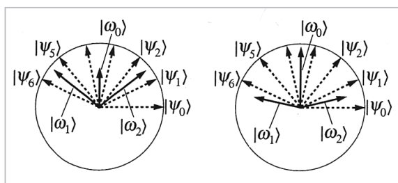
図3 7元信号の場合の最適測定ベクトル
