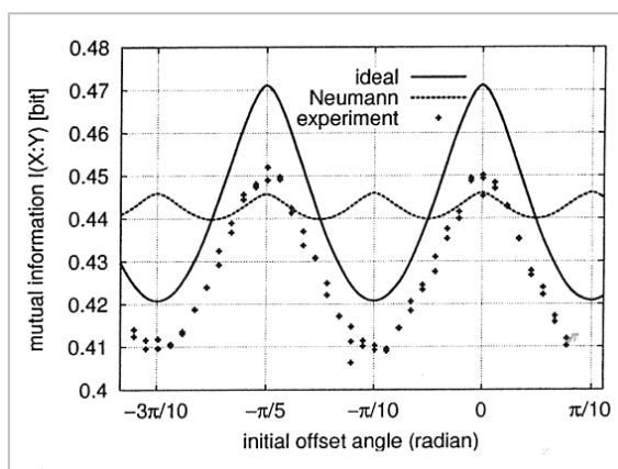
図10 5元信号の場合の相互情報量の \theta_0 依存性。 記号の定義は図8と同じ。
