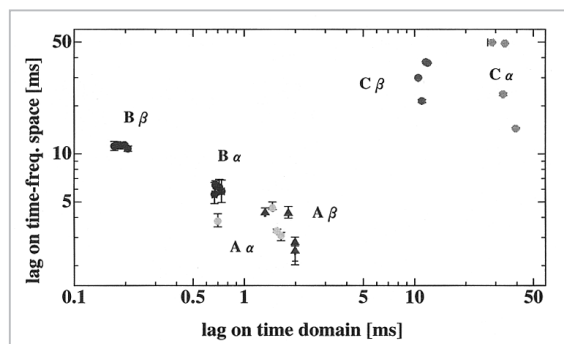
図5 立上り時、時間領域－時間周波数空間特徴量空間における無線機の分布
