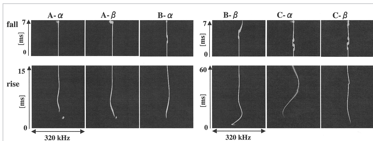
図3 無線機のモデルごとの立上り、立下り時間一周波数スペクトルパターン
