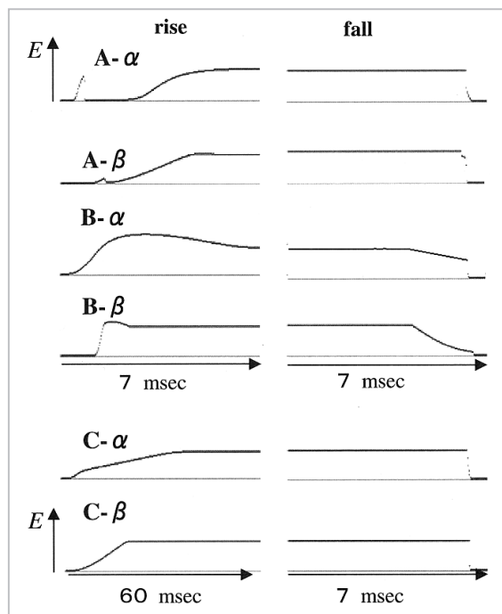
図1 無線機モデルごとの立上り、立下り振幅包絡線パターン
