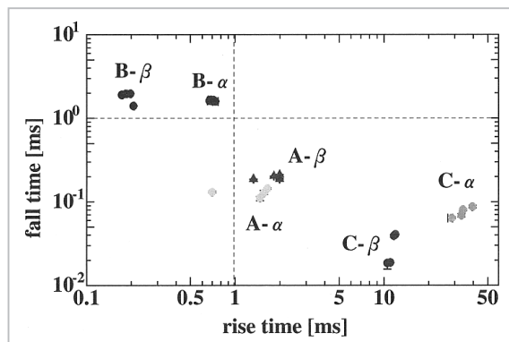
図2 立上り立下り時間特徴量空間における無線機の分布
