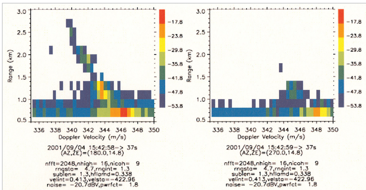
図4 RASS観測で取得したドップラスpekトルの距離速度断面図
