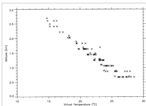
図5 10分間のRASS観測から得られた仮温度の高度分布
