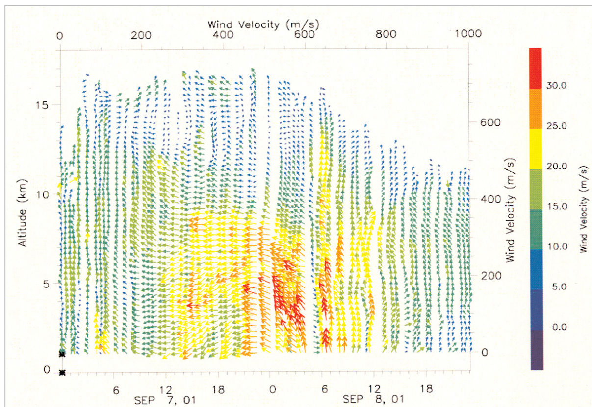
図3 400MHz帯ウィンドプロファイラによる水平風速ベクトルの30分平均値の時間高度分布
