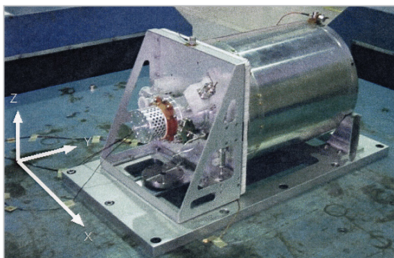
図6 振動試験の様子
