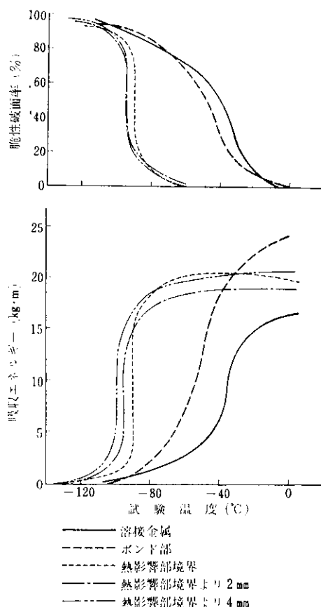
図 15 熱影響部の 2 mm V ノッチシャルビー 衝撃遷移曲線（5.0 mm 幅小型試験片）
