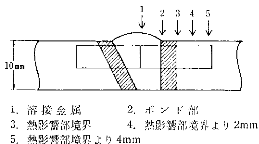
図 14 シャルビー衝撃試験片のノッチ位置
