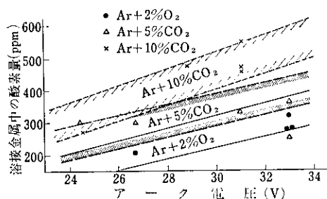
図 1 MIG 溶接金属中の酸素量とシールドガスの関係
