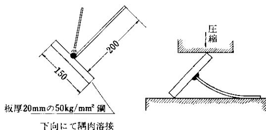
図 12 隅肉溶接曲げ試験片形状および曲げ試験方法
