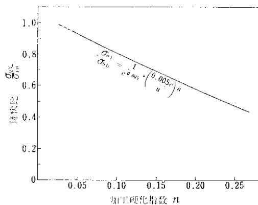
図 3 加工硬化指数と降伏比との関係
