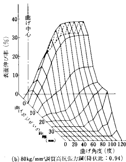
(b) 80kg/mm 2 調質高抗張力鋼(降伏比:0.94)
