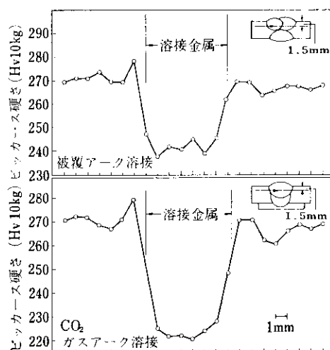
図 14 継手硬さ試験結果
