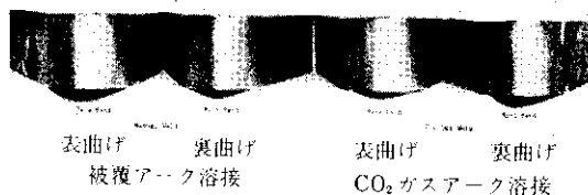
写真5 溶接継手曲げ試験結果
