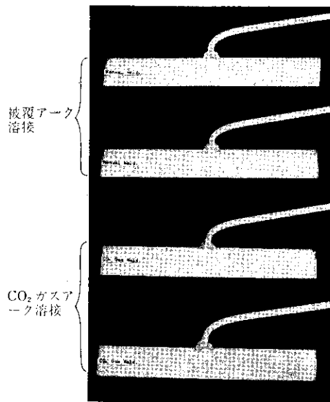
写真 3 隅肉溶接曲げ試験結果
