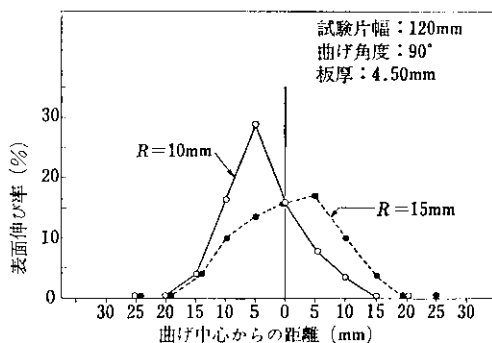
図 6 広幅曲げ試験による表面伸び率の分布 (HTP 80)
