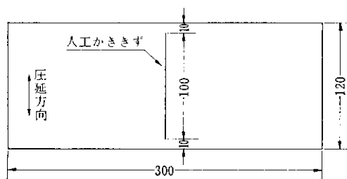
図8 人工かききずをつけた広幅曲げ試験片の形状
