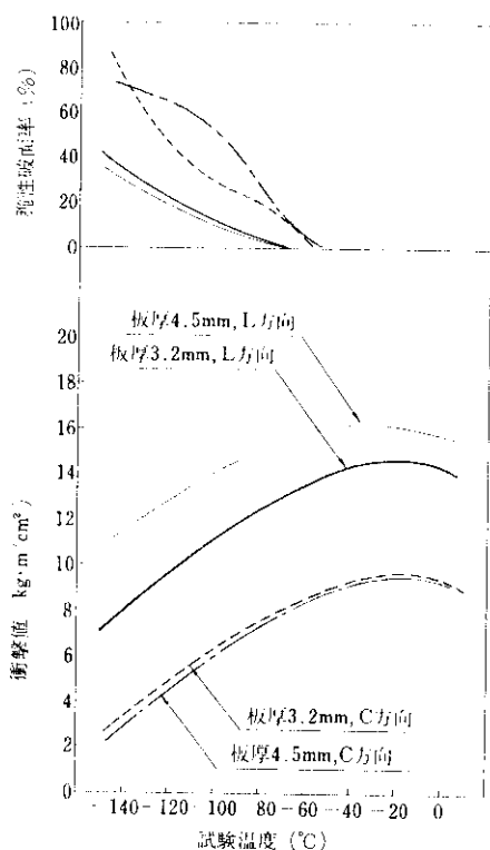
図 1 HTP 80 の 2mmV ノッチシャルピー衝撃試験結果
