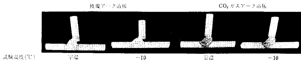
写真2 隅肉溶接拘束われ試験結果
