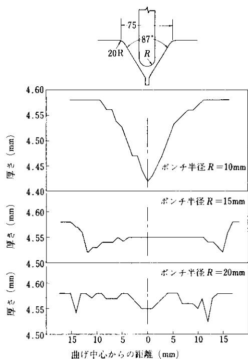
図 2 Vダイスを用いた曲げ加工による板厚の変化 (HTP 80, 板厚 4.58mm)
