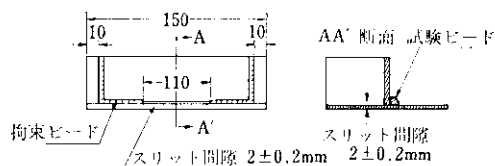
図11 隅肉溶接拘束割れ試験片形状
