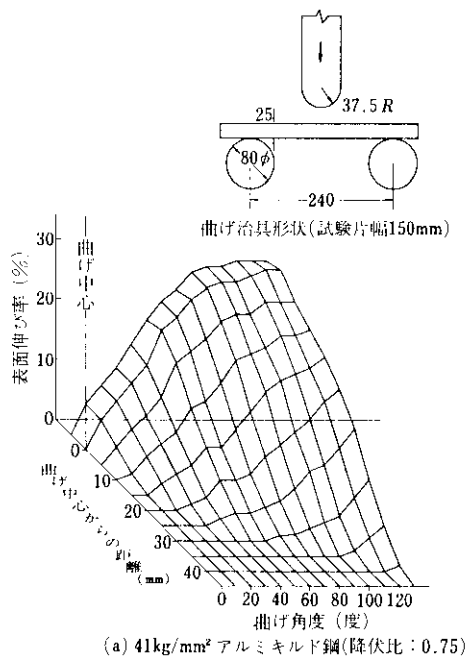
(a) 41kg/mm 2 アルミキルド鋼(降伏比:0.75)
