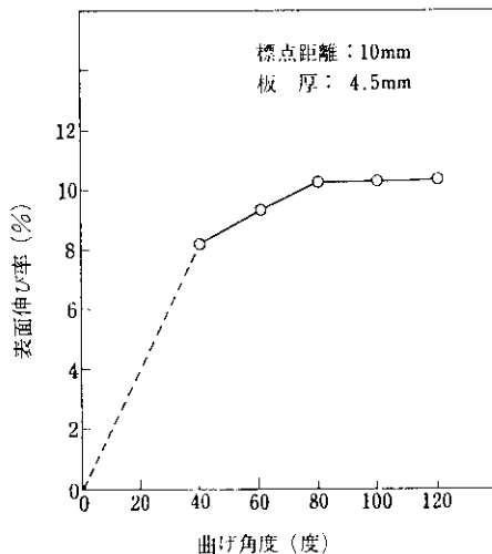
図10 溶接ビード曲げ試験治具による表面伸び率と曲げ角度との関係 (HTP 80)
