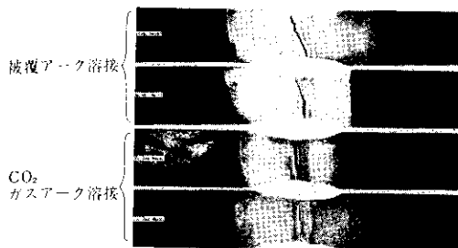
写真4 破断後の溶接継手引張試験片
