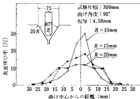
図 7 Vダイスによる曲げ加工時の表面伸び率の分布 (HTP 80)
