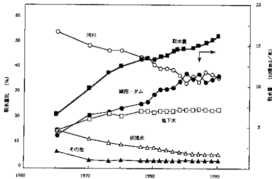
図1 水道水源取水量と水源の種類の変化
