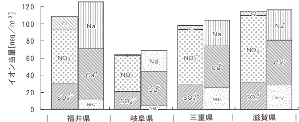
図6 平均粒径4.6 \mu\text{m} の当量比
