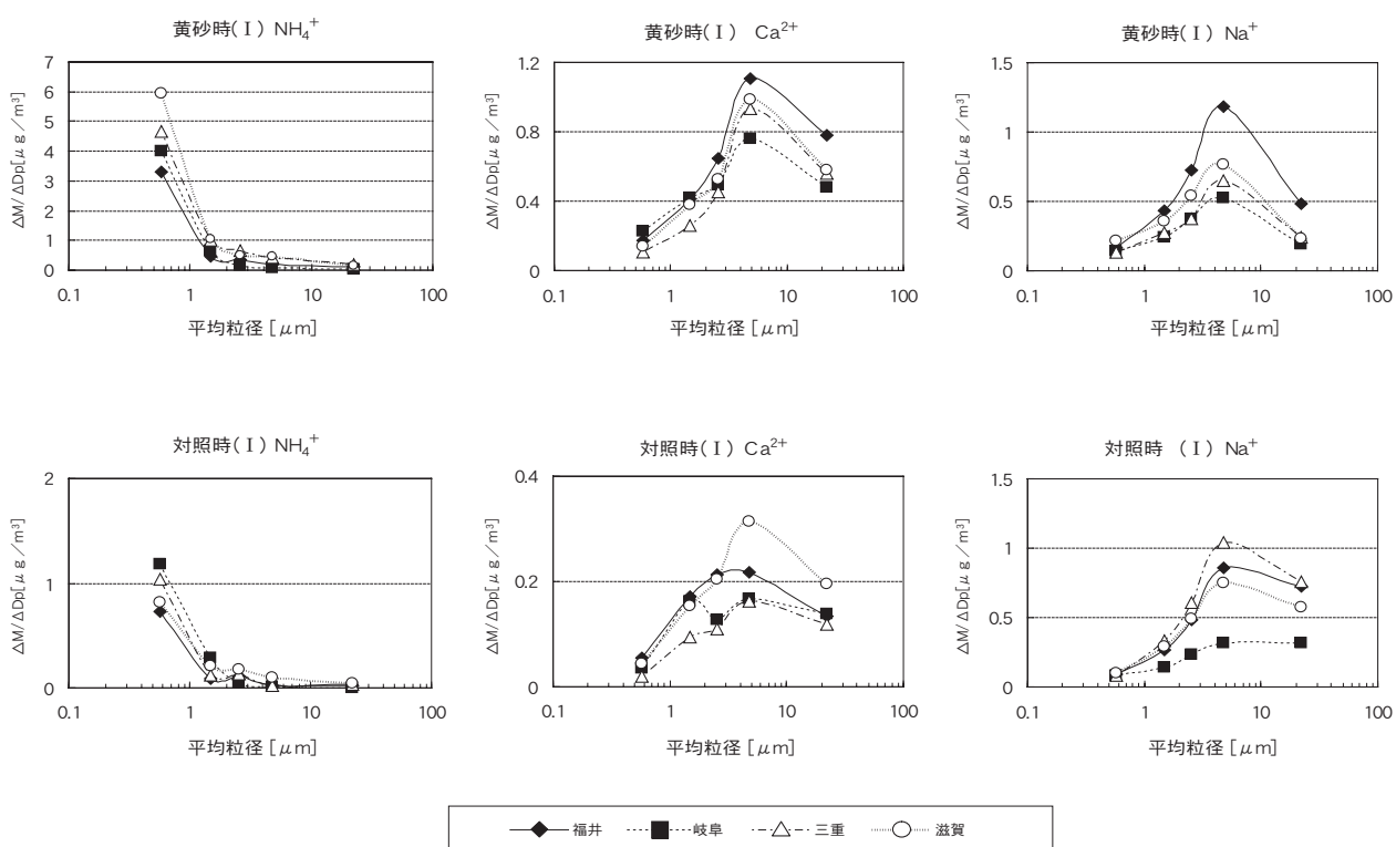
図4 各県における陽イオン成分
