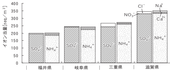
図5 平均粒径0.6 \mu\text{m} の当量比
