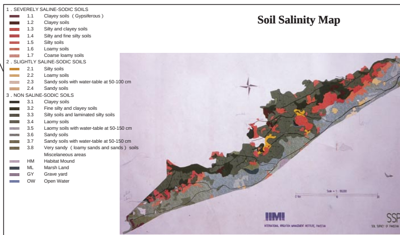
図4：土壌図 (Soil Salinity Map)
