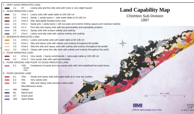
図3：土地利用図 (Land Capability Map)
