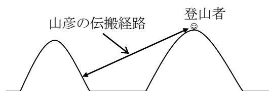
図5 山彦
