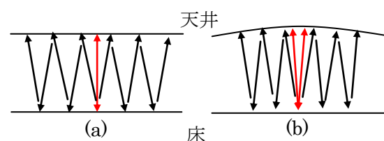
図6 鳴き竜
