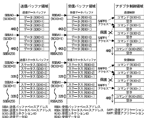
図3 アドレスマップ
