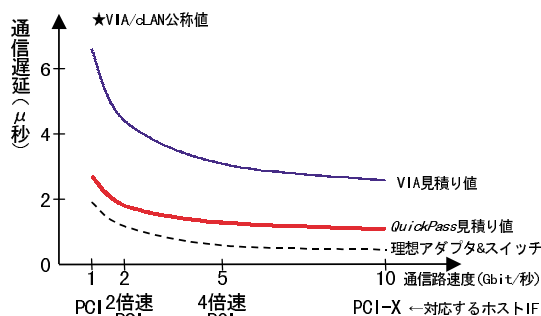
図 5 伝送速度と通信遅延の関係
