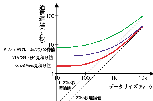
図 6 データサイズと通信遅延の関係
