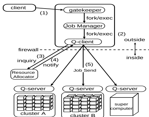
図 2 RMF の仕組みと動作の様子
