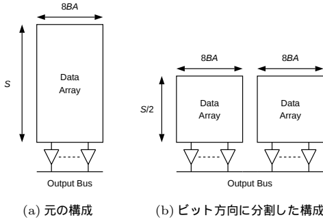
図 1 アクセス時間を削減するためのキャッシュの構成例
