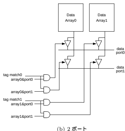
図2 出力回路
