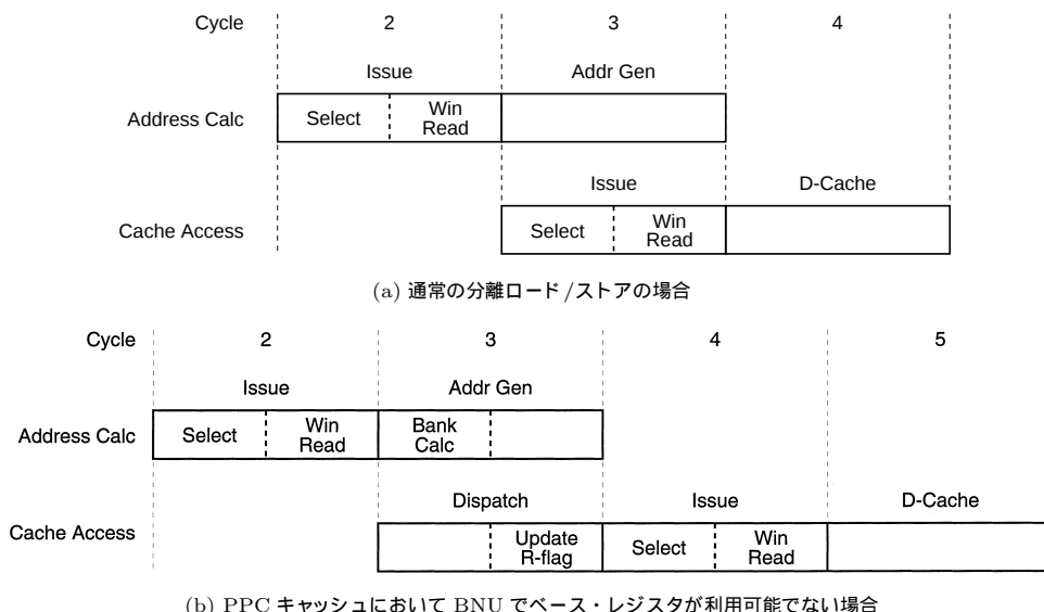
図 8 通常的分離ロード/ストアと PPC キャッシュにおける命令発行のタイミング
