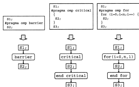
図6 OpenMP 指示文の並列フローグラフでの表現 Fig. 6 Representations of OpenMP directives in PFG.
