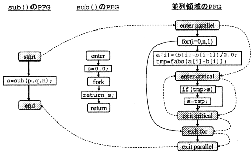
図 8 並列フローグラフと同期グラフ
