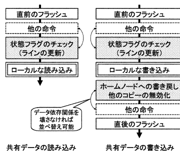
図 4 無効化プロトコルの動作
