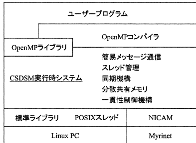
図 2 Omni/CSDSM の実行時システム
