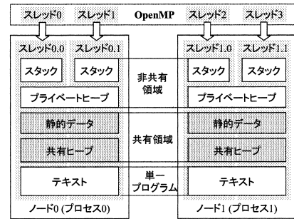
図 3 Omni/CSDSM の仮想アドレス空間
