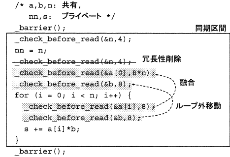
図 10 局所最適化
