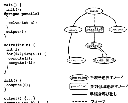
図 11 OpenMP プログラムとクローニング後のコールグラフ Fig. 11 An OpenMP program and its call graph after procedure cloning.
