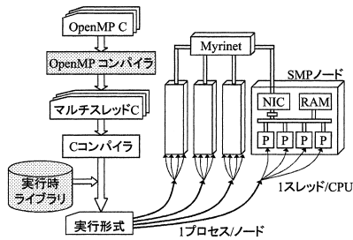
図 1 Omni/CSDSM のシステム構成
