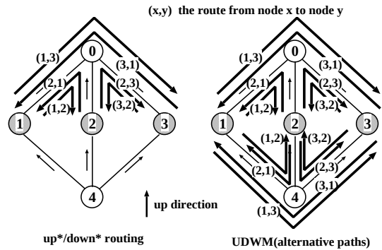
図3 5ノードのネットワークにおけるトラフィックの分散の比較 Fig. 3 An example of path distribution in the UDWM and up*/down* routing.
