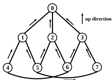
図1 BFS spanning treeに基づいた有向グラフ
