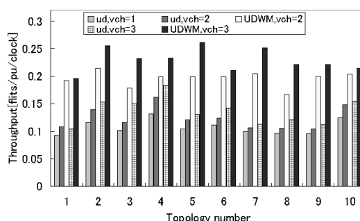
図 4 BFS, 16 ノードにおけるスループット
