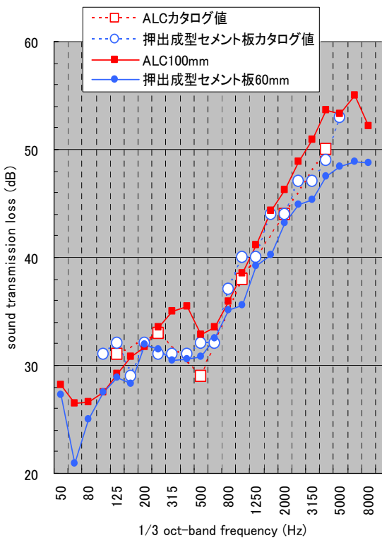
図-3 単体遮音性能の比較
