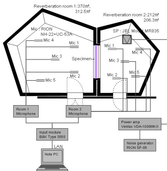
図－２ 測定ブロック図
