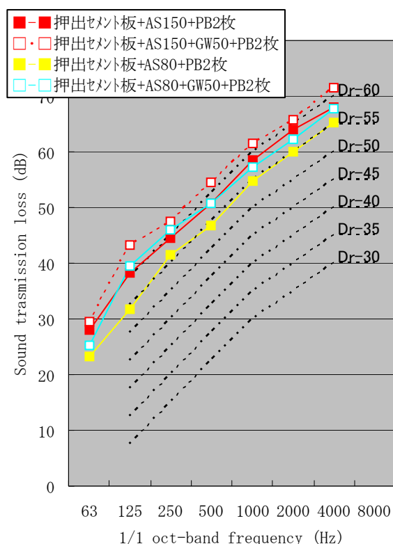
図-10 押出成型セメント板とPB2枚にGW挿入の効果
