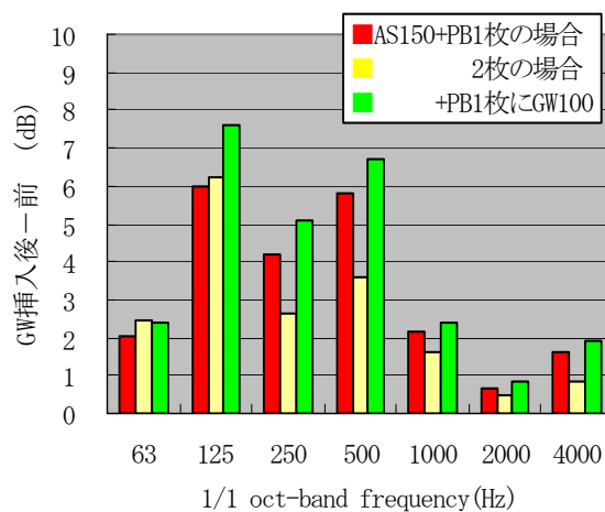
図－8 GW 挿入前後の差（ALC の場合）
