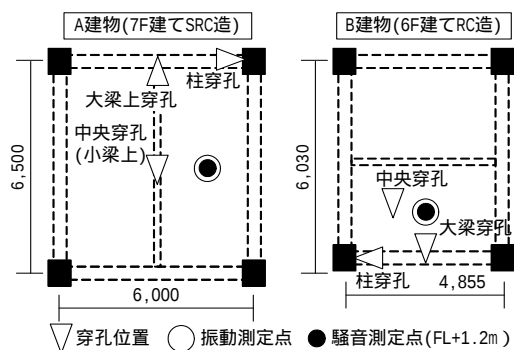
Fig. 1 穿孔位置と測定点
