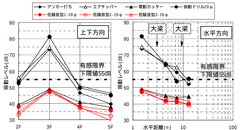
Fig. 7 振動レベルの上下と水平方向への伝搬(事例2) Propagation to a Vertical and Horizontal Direction
