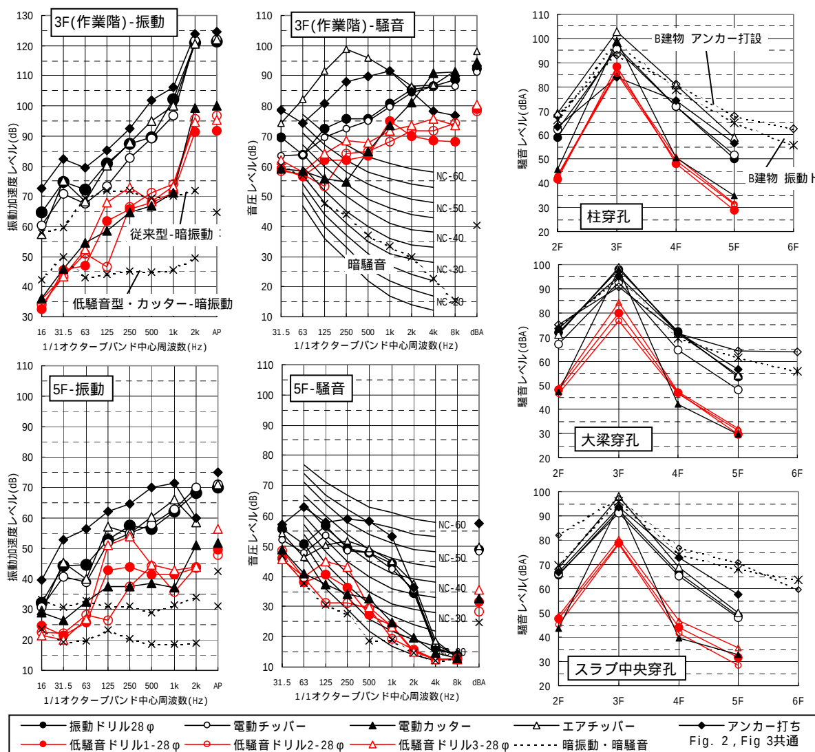
Fig. 2 各種工具の騒音・振動実測結果（柱作業時） Noise and Vibration (Working on Column)
