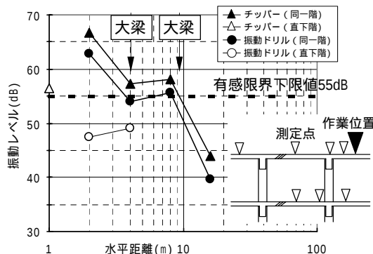
Fig. 5 振動レベルの距離減衰実測結果(事例1) Vibration Level Attenuation in Distance
