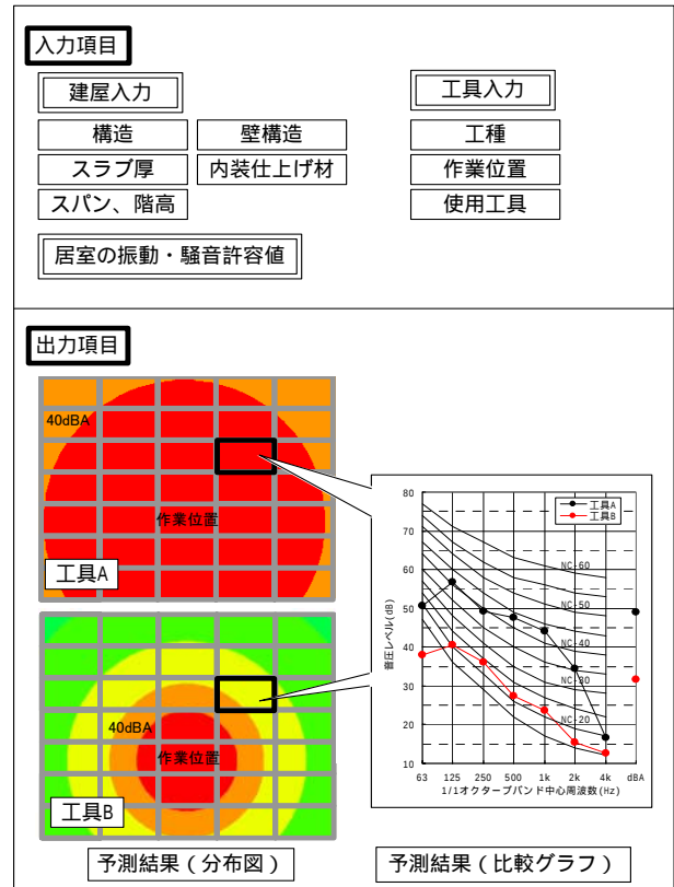
Fig. 9 予測システム入出力イメージ Image of System Input and Output
