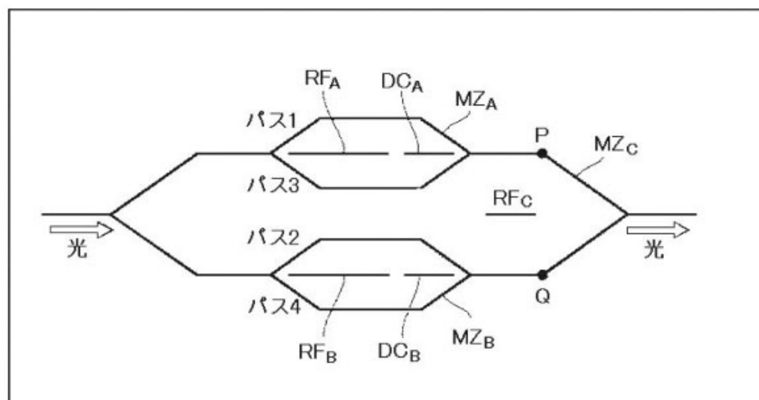
光 FSK 変調器の基本構成図
