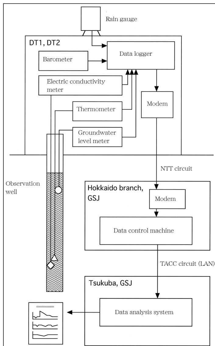
第4図 データの取得および流れ についての概略図.
