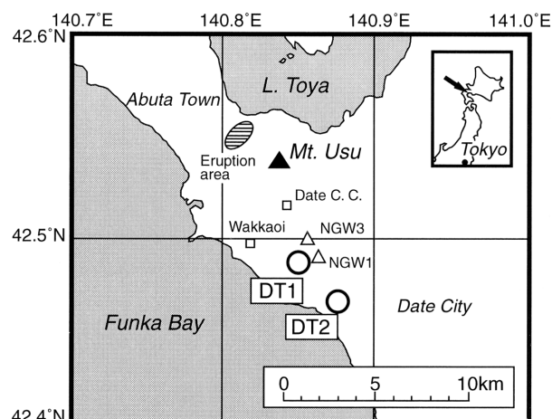
第1図 観測井DT1とDT2の位置. 四角印は1977年の噴火の際,地下水に \text{HCO}_3^- 濃度の上昇が観測された場所. 三角印は今回の噴火に伴って著しく動水位が変化した伊達市の水道ポンプ場.
