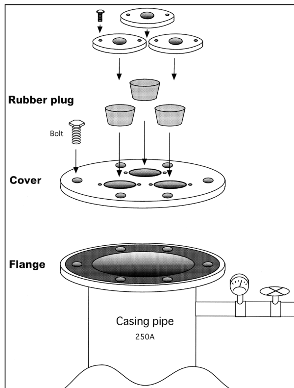
第3図 改造された孔口の構造。 Fig. 3 Repair of top of wells.
