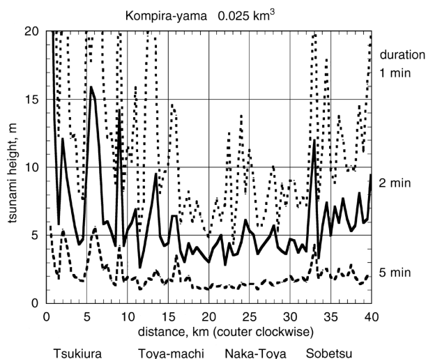
第3図 金比羅山の山体崩壊に伴う津波の高さ。継続時間1分間, 2分間, 5分間の3通りを示す。横軸は洞爺湖温泉町西端を起点に半時計回りに測ったキロ数で, 第1図の番号に対応する。
