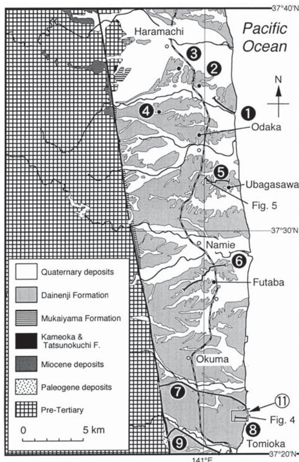
第3図 層序セクション作成位置図。久保ほか(1990, 1994, 2002)と柳沢ほか(1996)を基に作成。層序セクション; ●:小浜, ●:大甕, ●:大塚, ●:割羽迫, ●:水谷, ●:高瀬・渋川, ●:熊町-大川原, ●:小良ヶ浜, ●:本町西-上手岡河原沢, ⑪:小良ヶ浜北。
