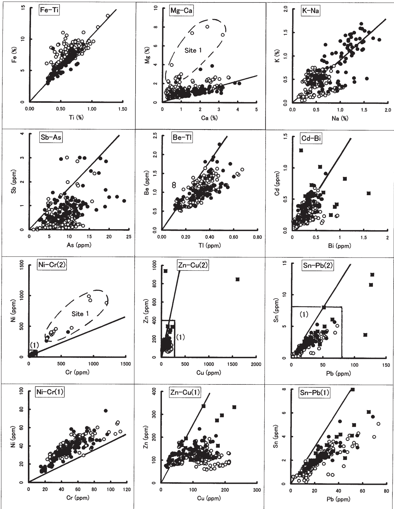
第5図 柱状試料(○), 表層試料(●), 東京東北部表層試料(■) 中元素濃度の比較. 直線は各元素の地殻存在比(Wedepohl, 1995).
