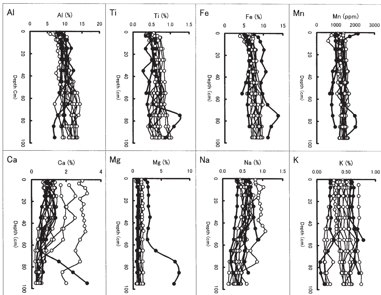
第2図 黒ボク土(○)と褐色森林土(●)柱状試料中主成分元素の鉛直濃度変化。
