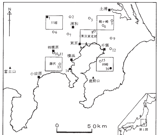
第1図 黒ボク土(○)と褐色森林土(●)柱状試料の採取地点と表層試料を採取した5地域(川越、龍ヶ崎、東京東北部、藤沢、姉崎)。
