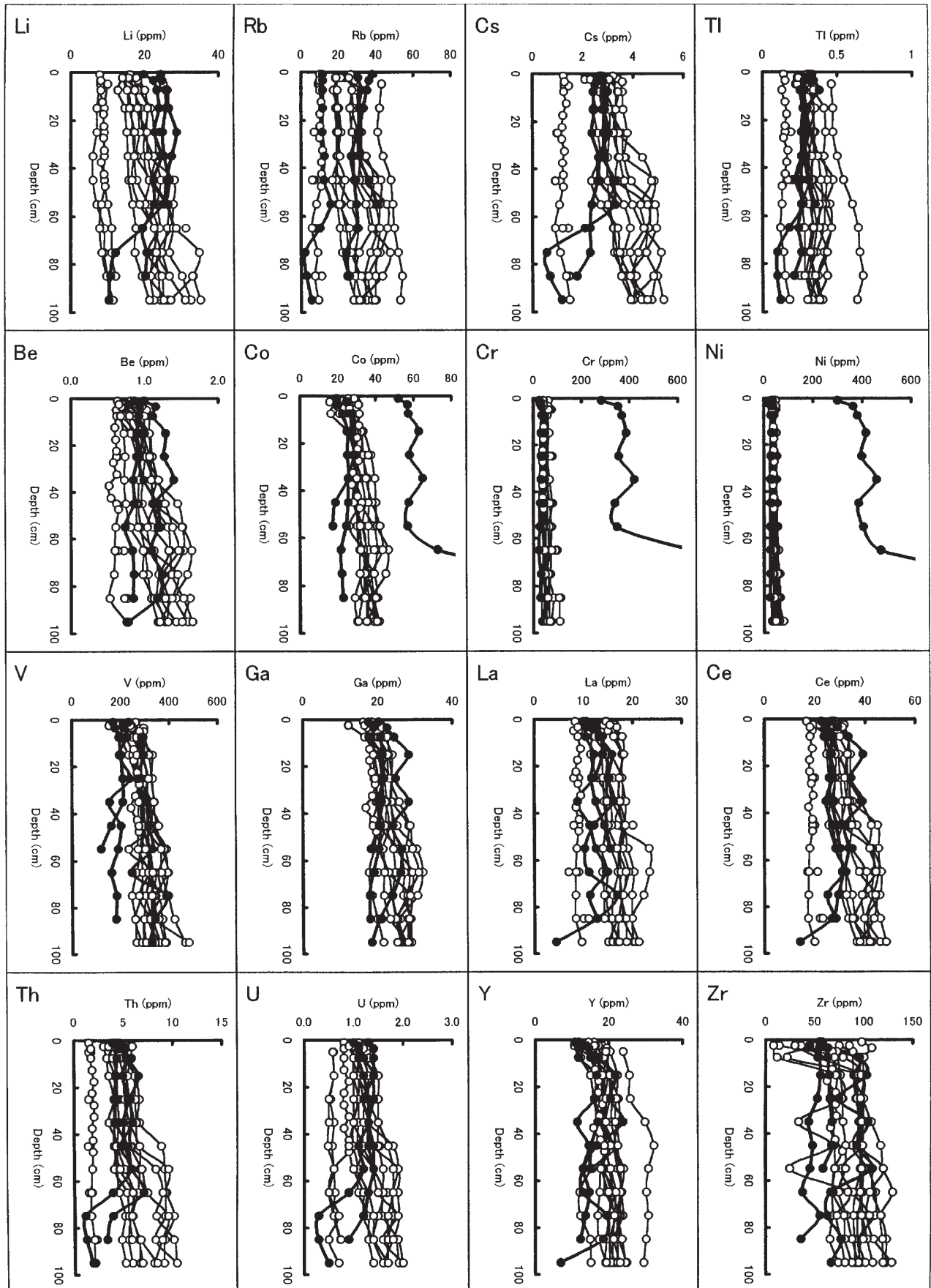
第4図 黒ボク土(○)と褐色森林土(●)柱状試料中微量元素の鉛直濃度変化(2).
