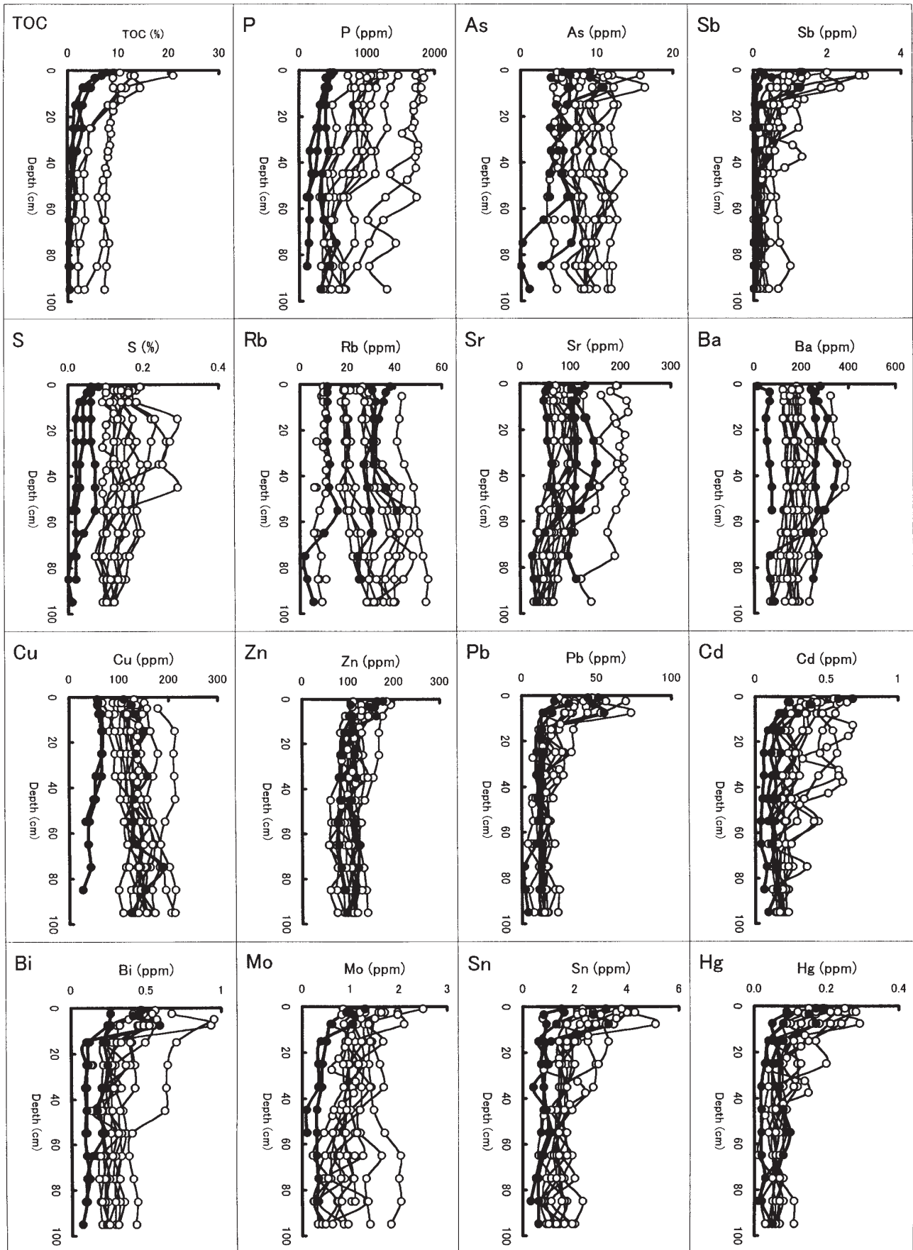
第3図 黒ボク土(○)と褐色森林土(●)柱状試料中微量元素の鉛直濃度変化(1).
