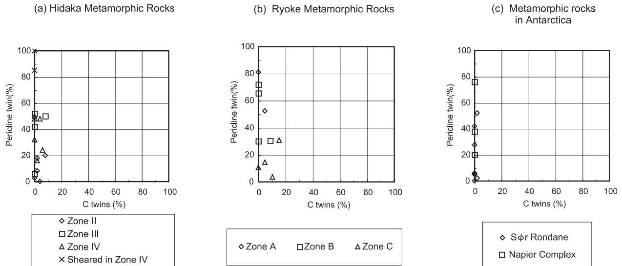
第2図 変成岩類の斜長石双晶頻度図
