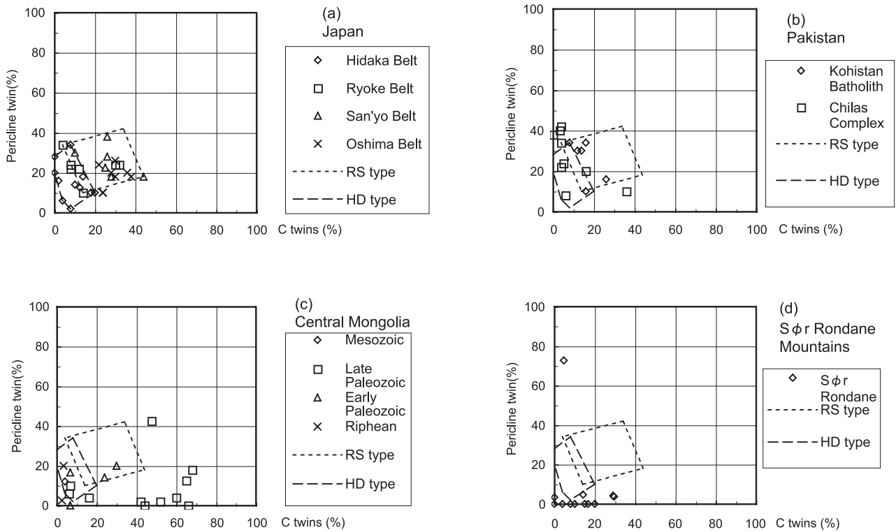
第1図 花崗岩類の斜長石双晶頻度図
