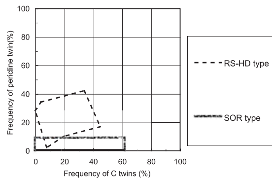
第3図 斜長石双晶に基づく花崗岩類識別図
