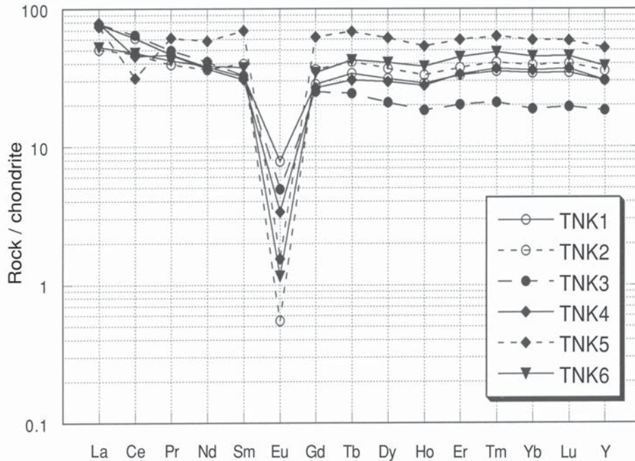
第2図 田上花崗岩の希土類元素の存在量 (コンドライト規格).
