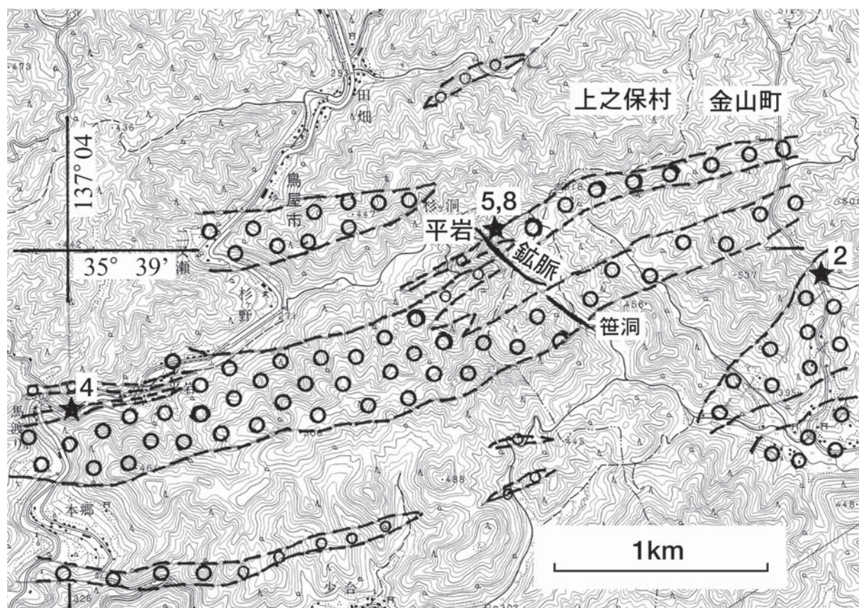
第2図 岐阜県、平岩鉱床付近の花崗斑岩類(○印部)の分布 (五十嵐, 1959 を簡略化). ★に番号は第2表の分析試料位置.
