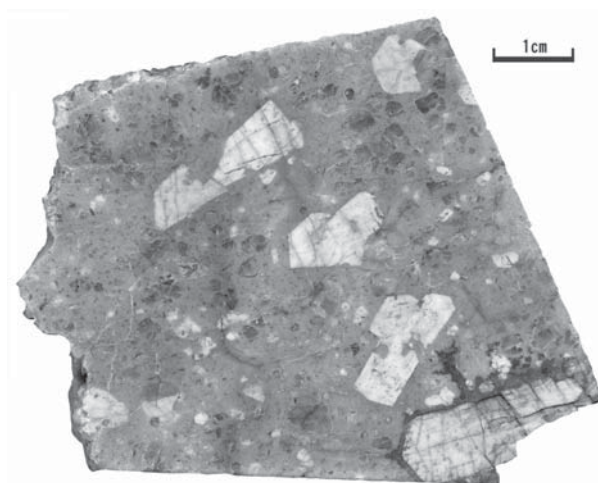
第4図 バイカル湖南部の高フッ素花崗斑岩の外観.
