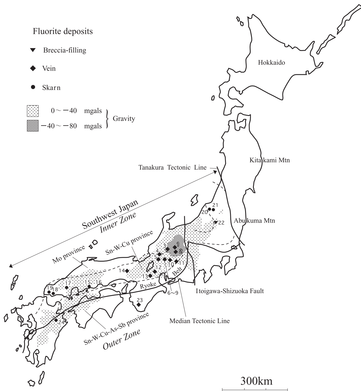
第1図 日本のほたる石鉱床の分布とブーゲ異常から推定される地殻の厚さ (石原・寺島, 1977b, Fig. 3 に加筆). 番号は第1表のものと一致する.
