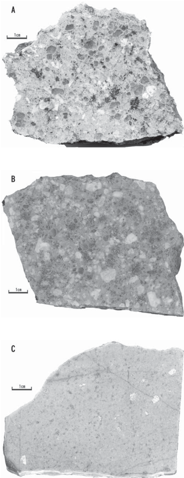
第3図 平岩地区、ほたる石鉱床に関係する岩脈類の外観。 A. 最も新鮮な花崗斑岩 (HWA2). B. 弱変質花崗斑岩 (HWA5). 長石斑晶の輪郭がぼけている. C. 変質フェルサイト (HWA8).
