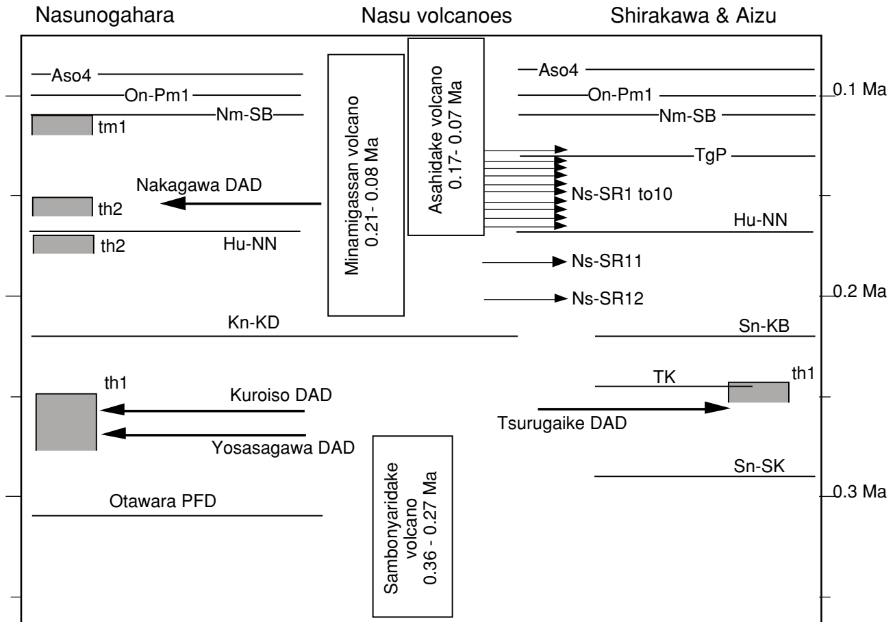
第7図 那須火山群，岩屑なだれ堆積物及び指標テフラ層の層序関係。Aso4 = Aso4 テフラ，Hu-NN = 燧ヶ岳・七入テフラ，Kn-KD = 鬼怒沼・黒田原テフラ，Nm-SB = 沼沢・芝原テフラ，Ns-SR1 to 12 = 那須・白河1～12 テフラ群，On-Pm1 = 御岳・Pm1 テフラ，Sn-KB = 砂子原・久保田テフラ，Sn-SK = 砂子原・佐賀瀬川テフラ，TgP = 田頭テフラ，TK = 高杖テフラ，DAD = 岩屑なだれ堆積物，PFD = 火砕流堆積物，th1 = 高位I段丘堆積物，th2 = 高位II段丘堆積物，tm1 = 中位I段丘堆積物。山元 (1999b) を一部改変。
