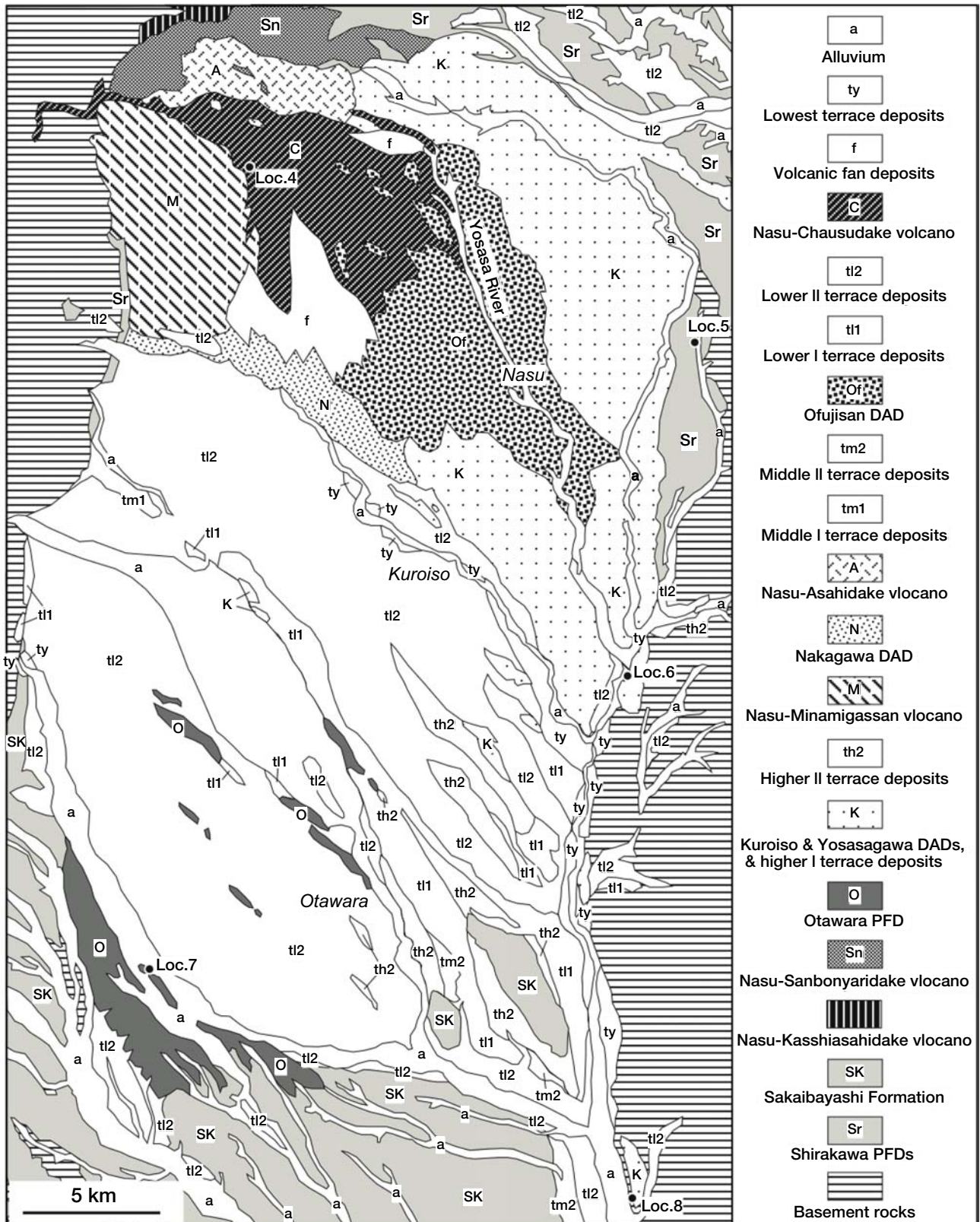
第4図 那須火山群及び那須野が原扇状地周辺の第四紀層地質図。DAD＝岩屑なだれ堆積物、PFD＝火砕流堆積物。位置は第1図を参照のこと。
