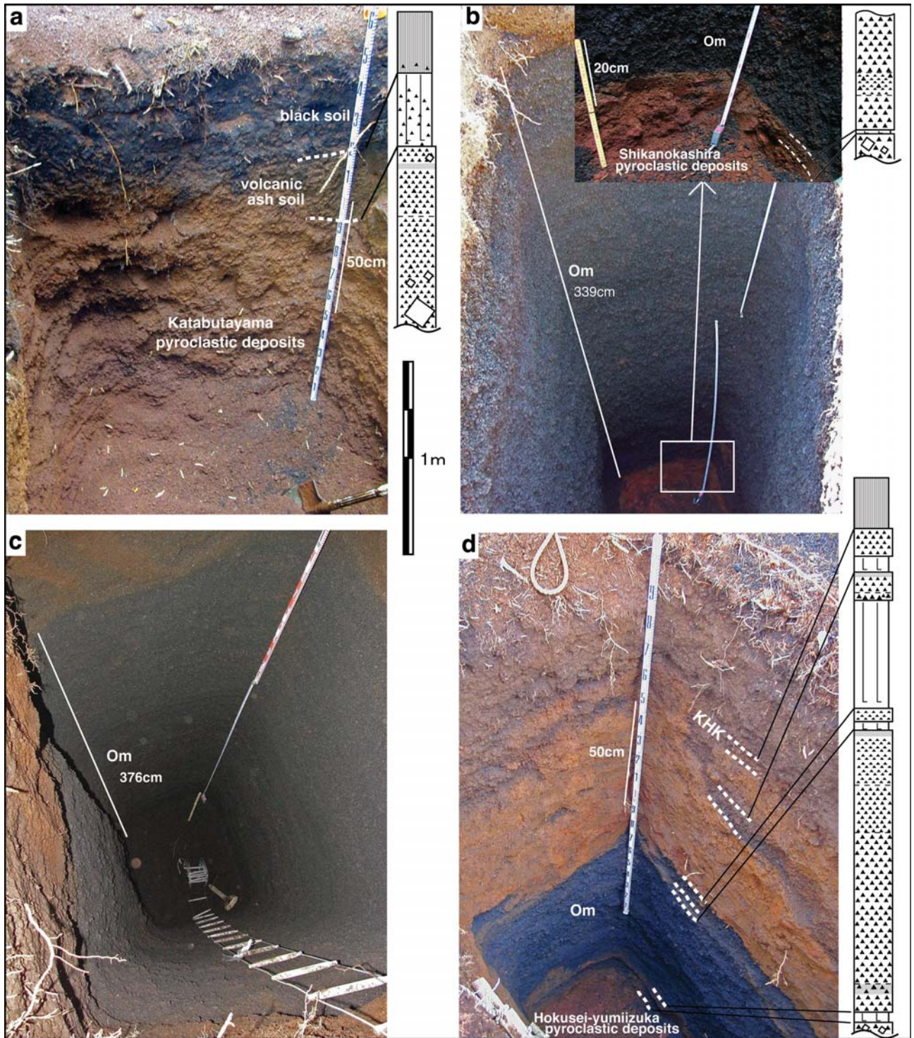
第3図 トレンチ写真と柱状図. 片蓋山 (a), 鹿の頭 (b), 榎尾山 (c), 北西弓射塚 (d) の各スコリア丘. 凡例は第2図と同じ. Fig. 3 Photographs and column sections of the Katabutayama (a), Shikanokashira (b), Tsugaoyama (c), and Hokusei-yumiizuka (d) scoria cones. Symbols are same with those in Fig. 2.
