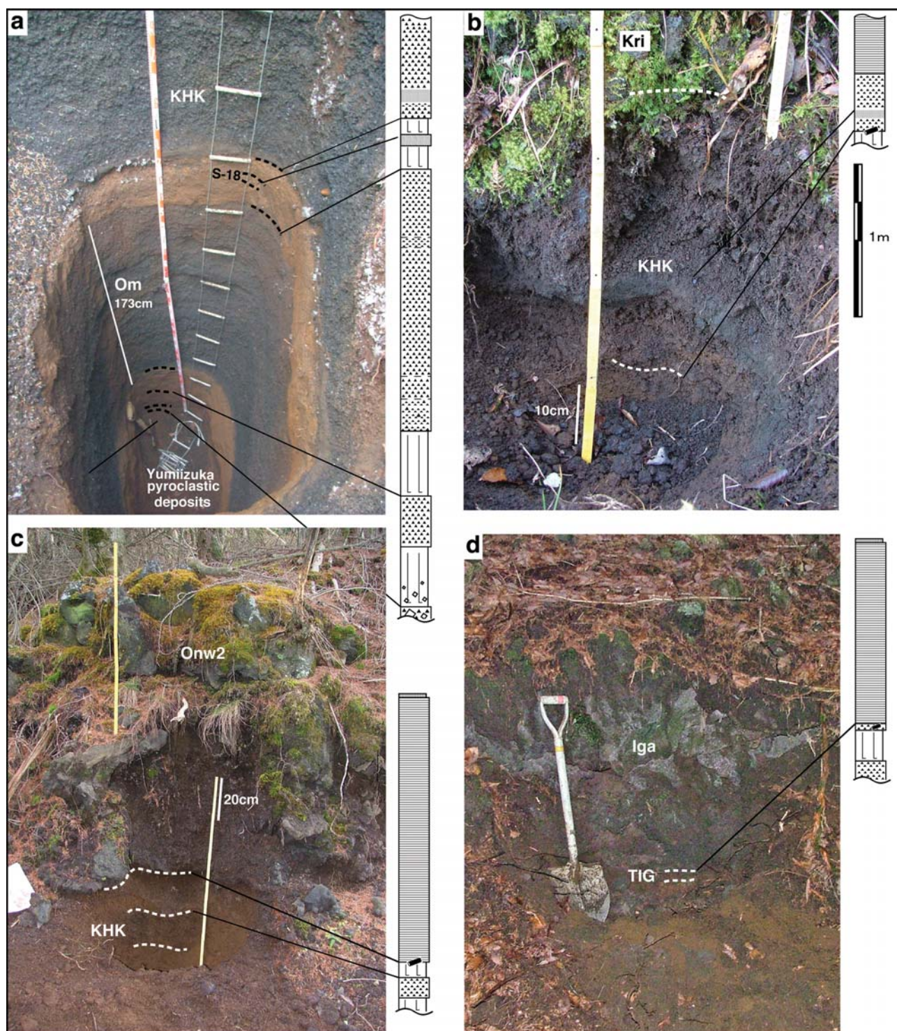
第4図 トレンチ及び露頭写真と柱状図. 弓射塚スコリア丘 (a), 露頭 Loc.1 (b), 露頭 Loc.2 (c), 露頭 Loc.3 (d) の各スコリア丘. 凡例は第2図と同じ.
