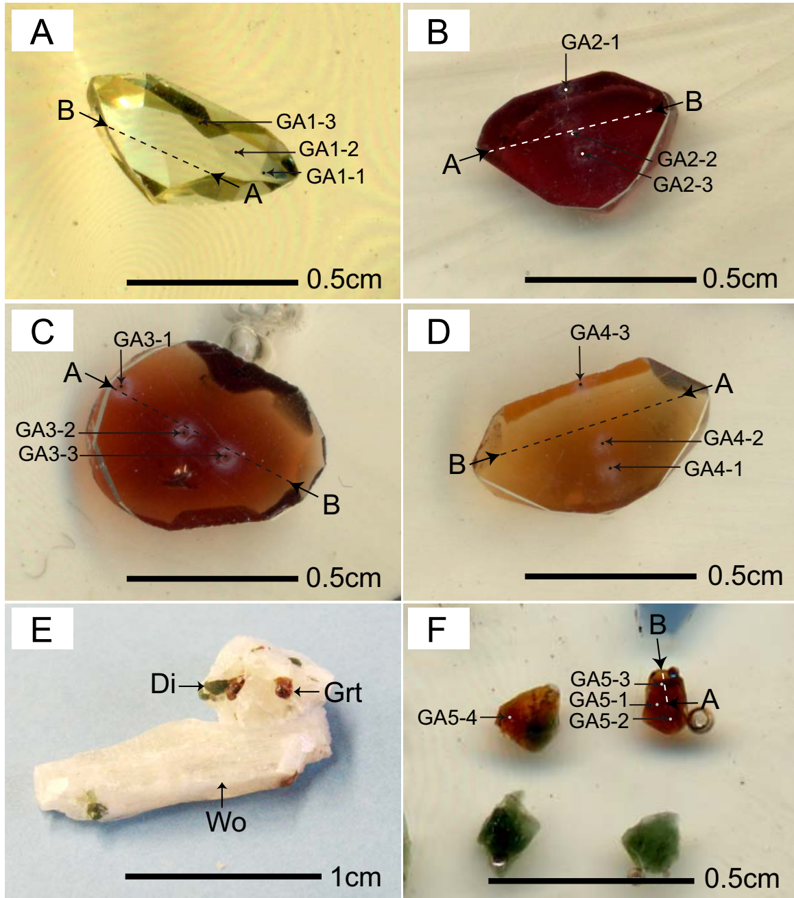
第1図 琢磨した分析試料のスカン画像とGA5のサンプル写真. (A) GA1. (B) GA2. (C) GA3. (D) GA4. (E) GA5のサンプル写真. ザクロ石 (Grt) は透輝石 (Di) とともに珪灰石 (Wo) 中に産する. (F) GA5.
