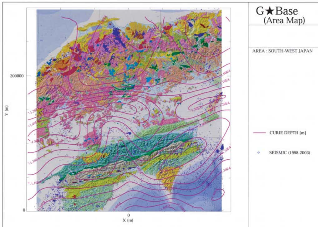
第14図 中国・四国地方の地質図、震源分布、キュリー点等温面深度分布の対比(震源は標高0～20 kmレベルで発生したものをプロット)。
