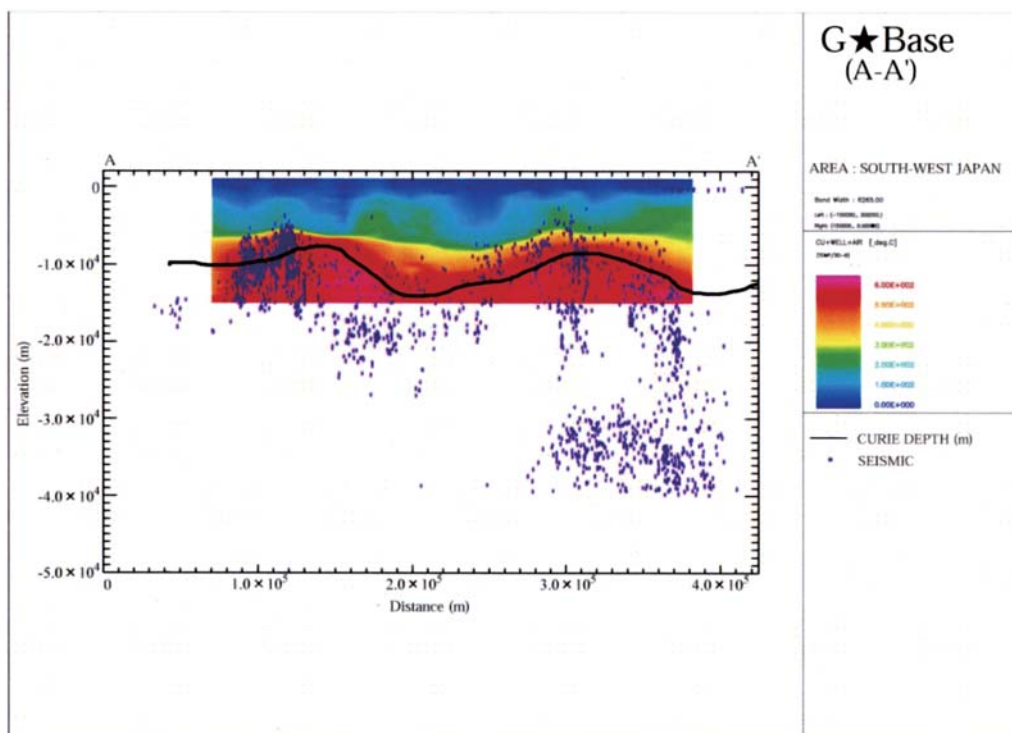
第 18 図 中国・四国地方の温度、震源分布及びキュリー点等温面深度分布の対比（第 3 図 A-A' 断面）（震源は断面線の両側 20 km の幅で発生したものを投影）。
