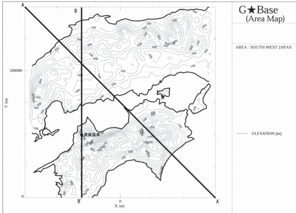
第 3 図 研究対象地域と断面位置（中国・四国地方）.
