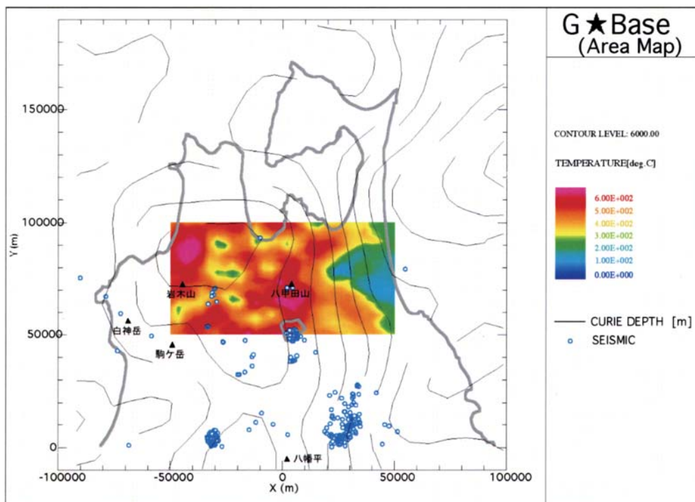
第10図 東北地方北部の温度(標高-6km), 震源分布及びキュリー点等温面深度分布の対比(震源は表示標高の±2kmで発生したものをプロット)。
