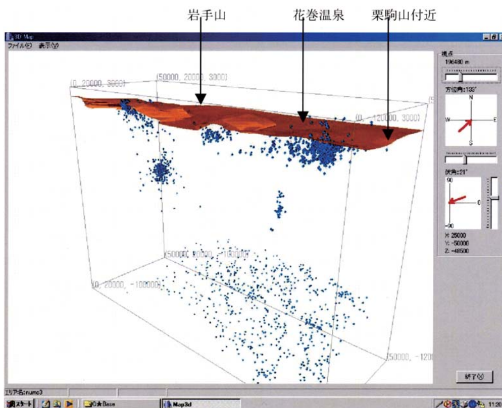
第 8 図 東北地方中北部の花巻温泉付近を通る南北断面（第 1 図 B-B' 断面）の地下 100 km までの三次元分布図（500 °C 等面温面と震源分布）（南西上方から）。
