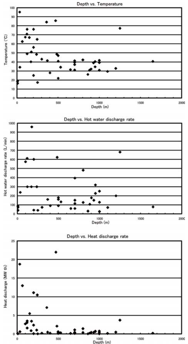
第2図 中国地域の深度 - 温度, 深度 - 湧出量, 深度 - 放熱量の関係。
