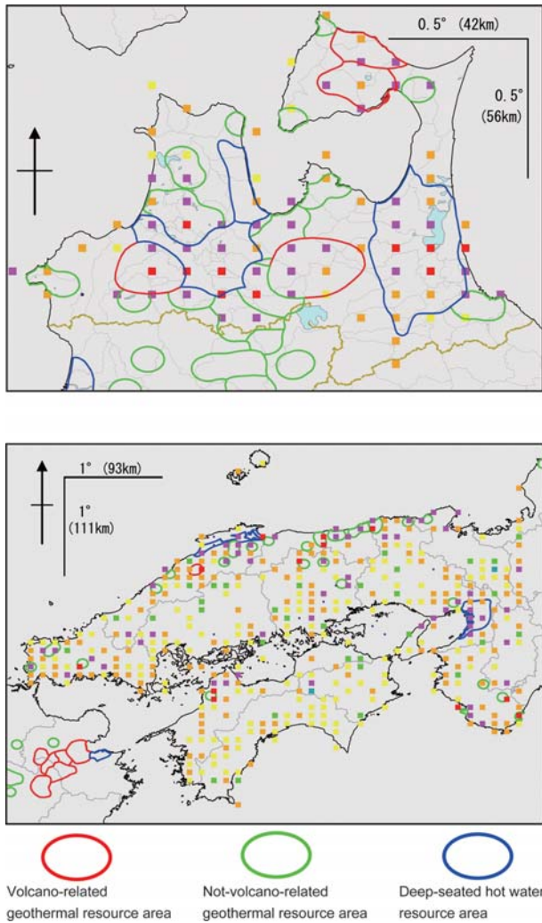
第5図 青森地域と中国・四国地域の温泉放熱量分布と地熱資源図（阪口・高橋，2002）による地熱資源賦存地域。
