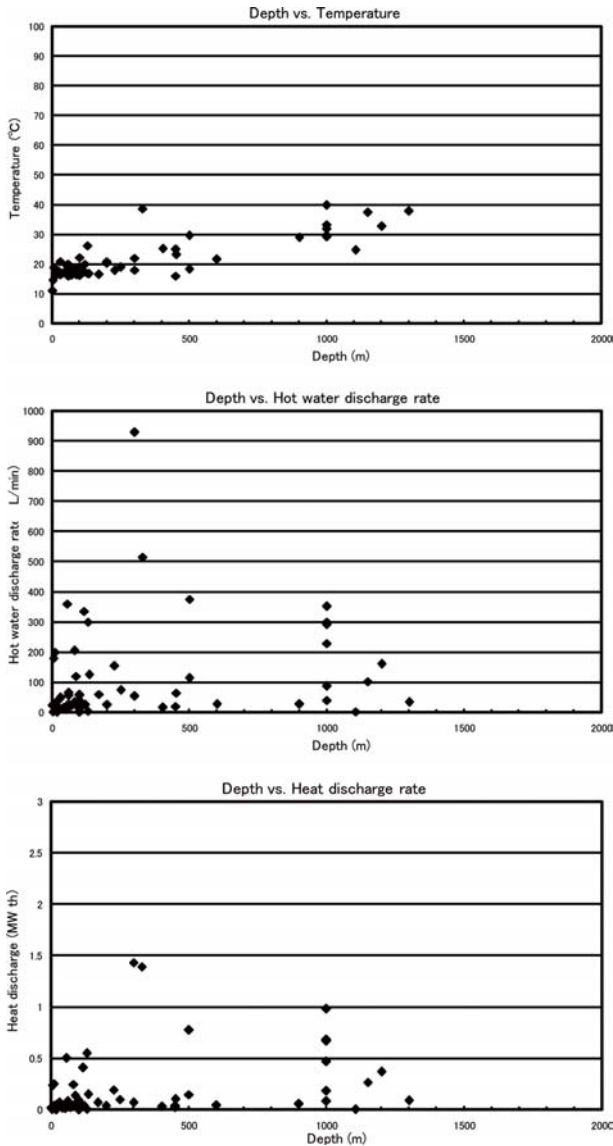
第3図 四国地域の深度 - 温度，深度 - 湧出量，深度 - 放熱量の関係。
