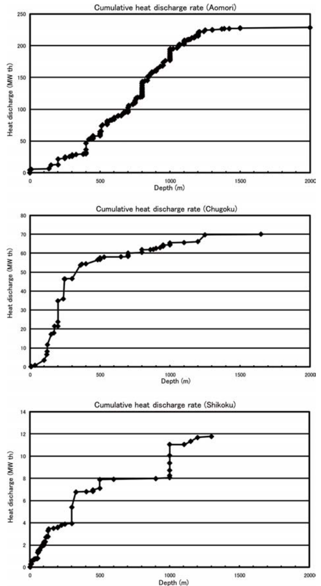
第4図 各地域の深度方向への放熱量の累計。
