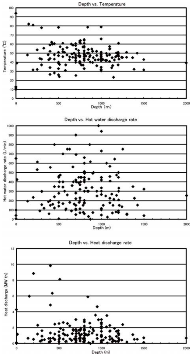
第1図 青森地域の深度 - 温度, 深度 - 湧出量, 深度 - 放熱量の関係。
